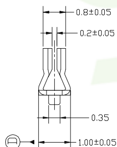
A-A SEC
