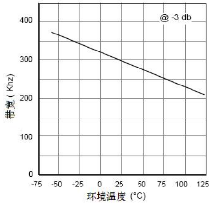
图 3. 带宽与温度的关系
