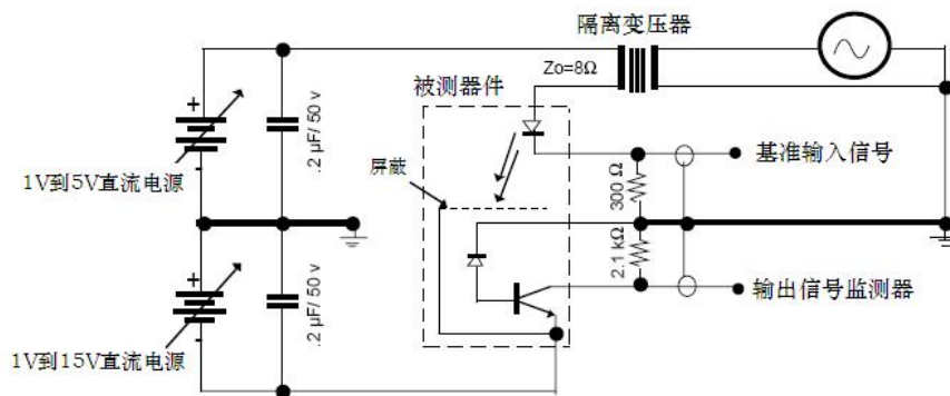
图 4. 增益和带宽测试电路
