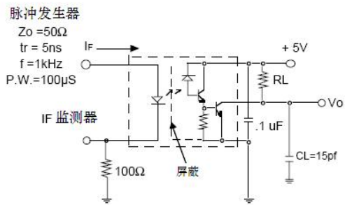
图 5. 开关测试电路
