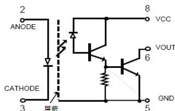
电原理图
