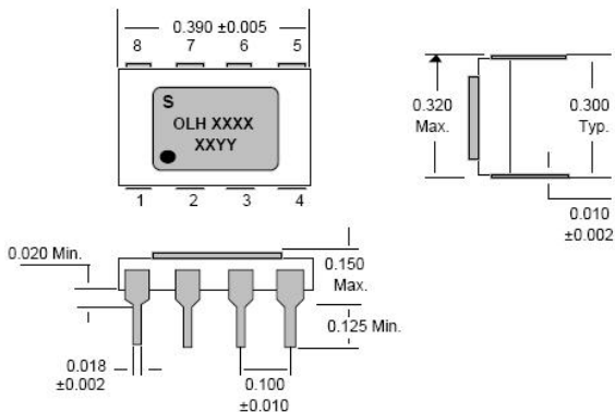
封装外形图
