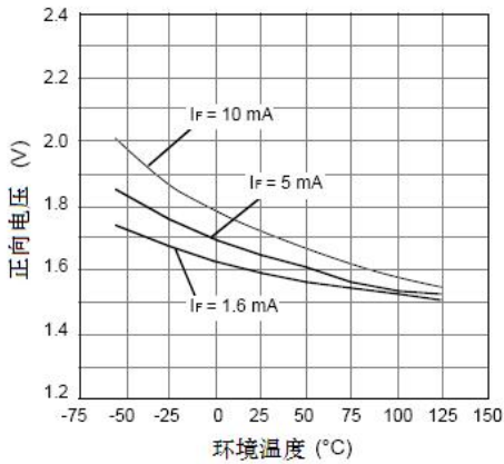
图 1. LED 的正向特性
