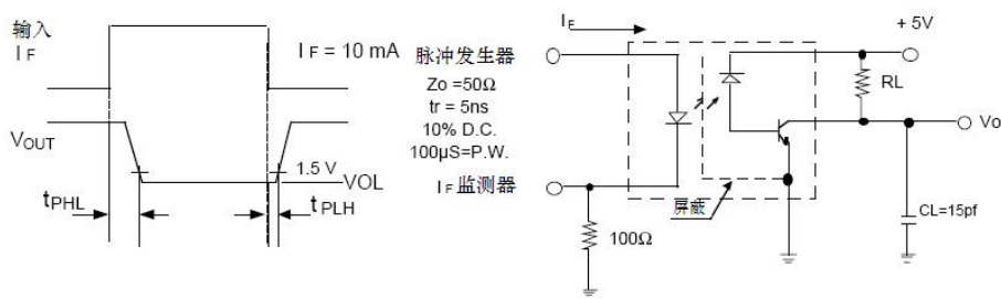
图 4. 开关测试电路
