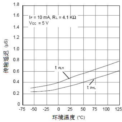
图 3. 传输延迟与温度的关系
