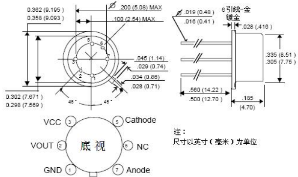
封装外形图
