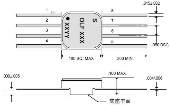
封装外形图
