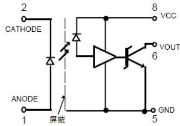
电原理图
