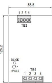
前视图
