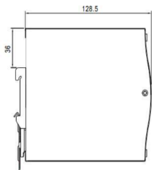
侧视图
