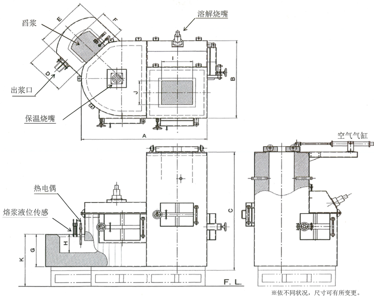
SER (露米美特) 炉尺寸表
