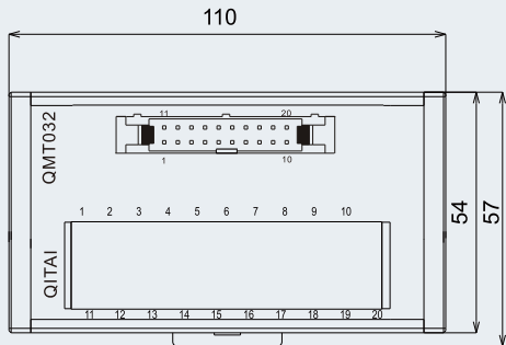
外形图 Dimensions
