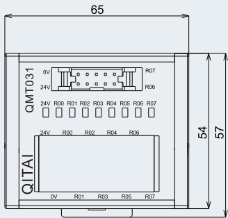
外形图 Dimensions
