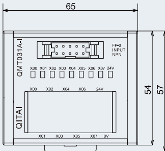
外形图 Dimensions
