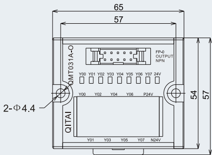
外形图 Dimensions
