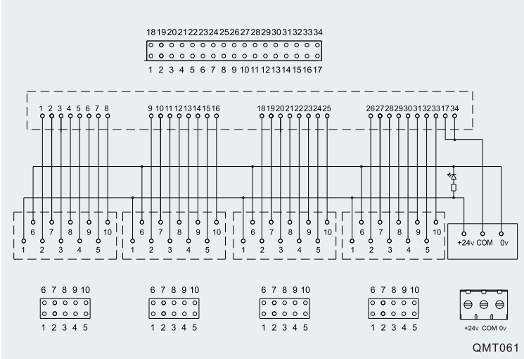
配线图 Wiring Diagram
