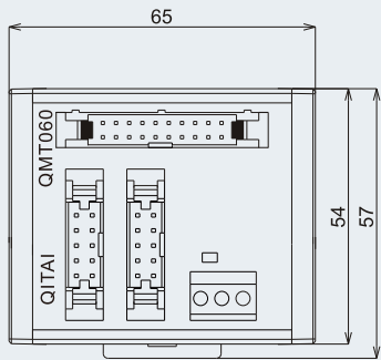
外形图 Dimensions
