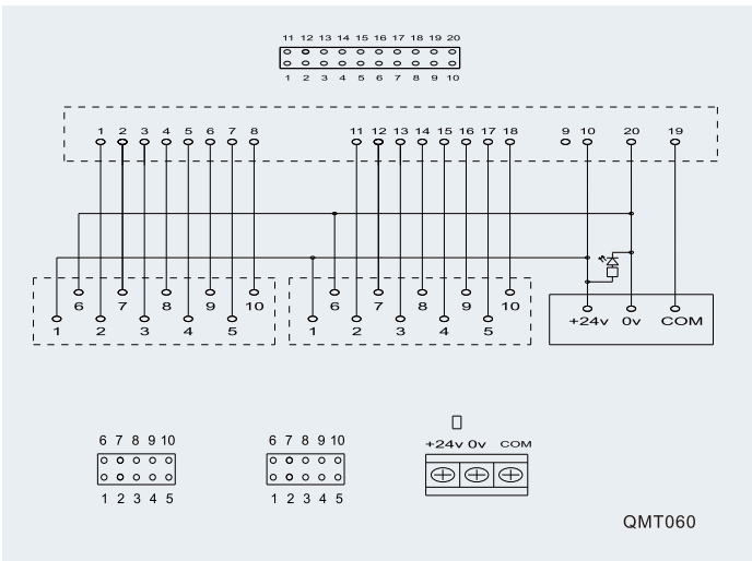
配线图 Wiring Diagram
