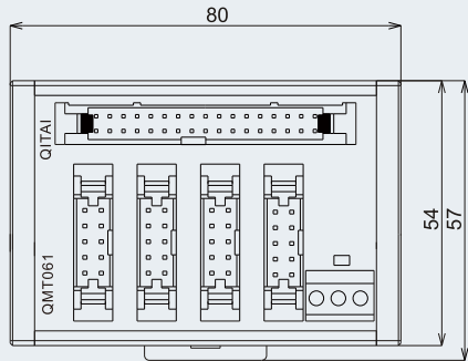
外形图 Dimensions
