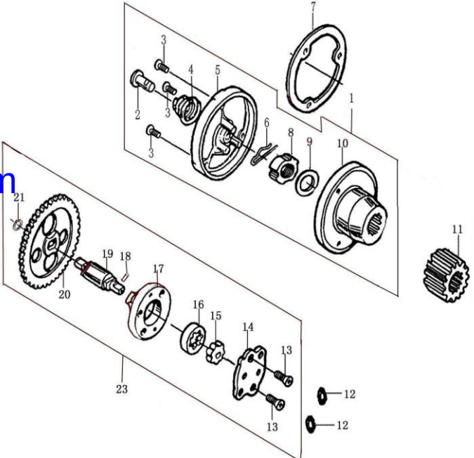
机油泵部件/机油滤清器部件 OIL PUMP/OIL FILTER
