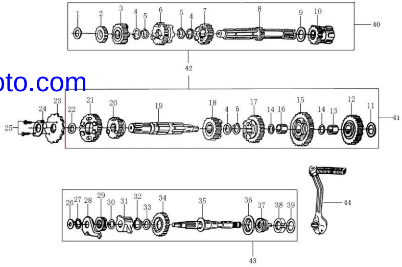
传动机构 TRANSMISSION MECHANISM
