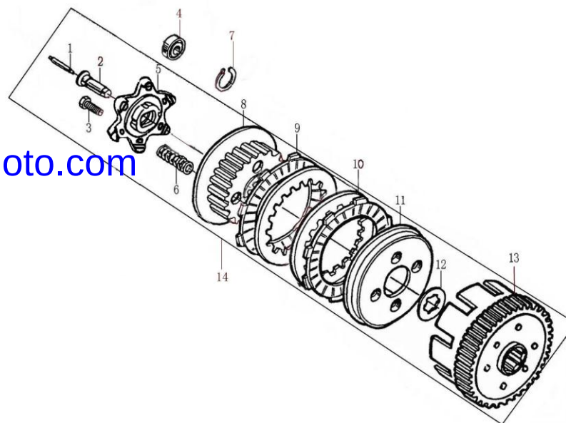
离合器总成 CLUTCH ASSY
