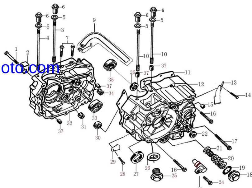
曲轴箱 CRANKCASE
