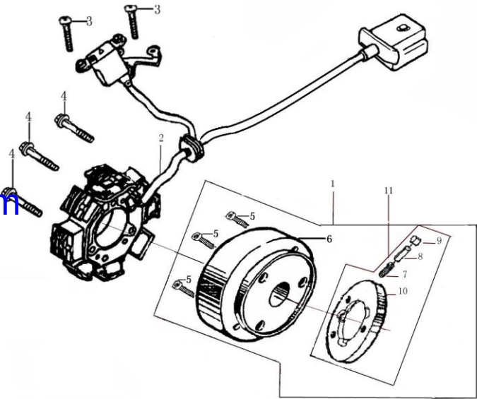
磁电机总成 MAGNETO COMP
