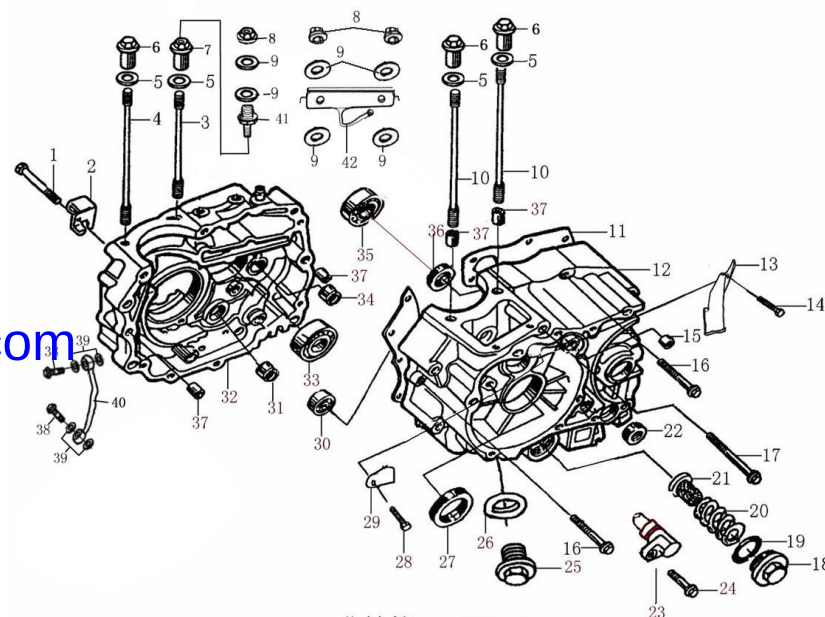
曲轴箱 CRANKCASE
