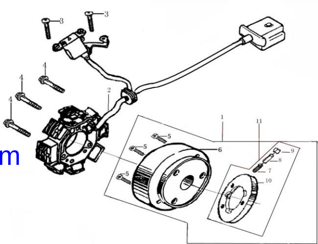
磁电机总成 MAGNETO COMP
