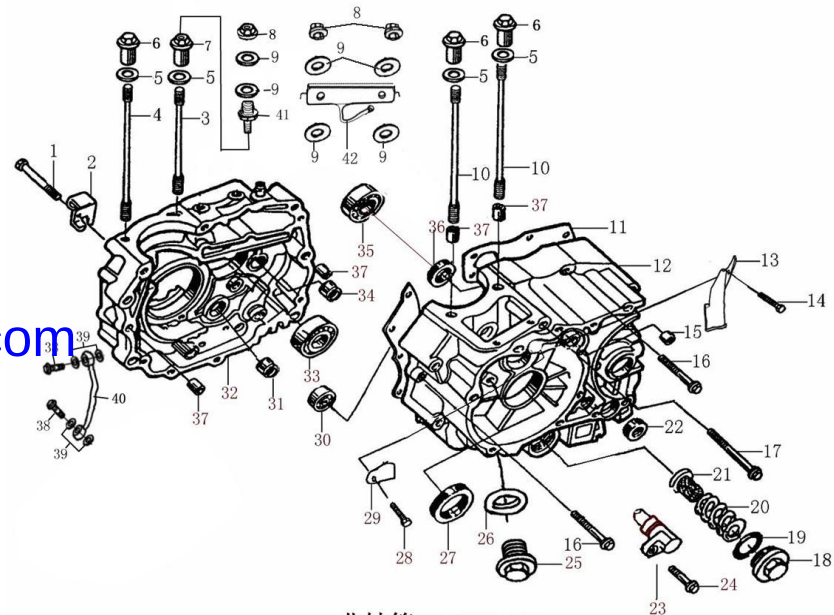
曲轴箱 CRANKCASE
