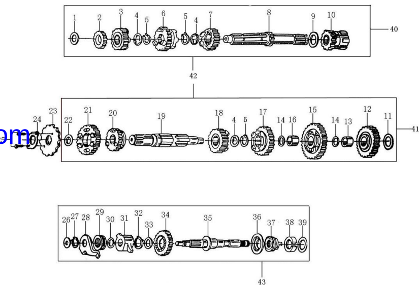
传动机构 TRANSMISSION MECHANISM
