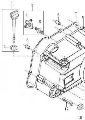
右曲轴 RIGHT CRANK
