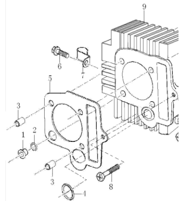
气缸体部件 CYLINDER ASSY
