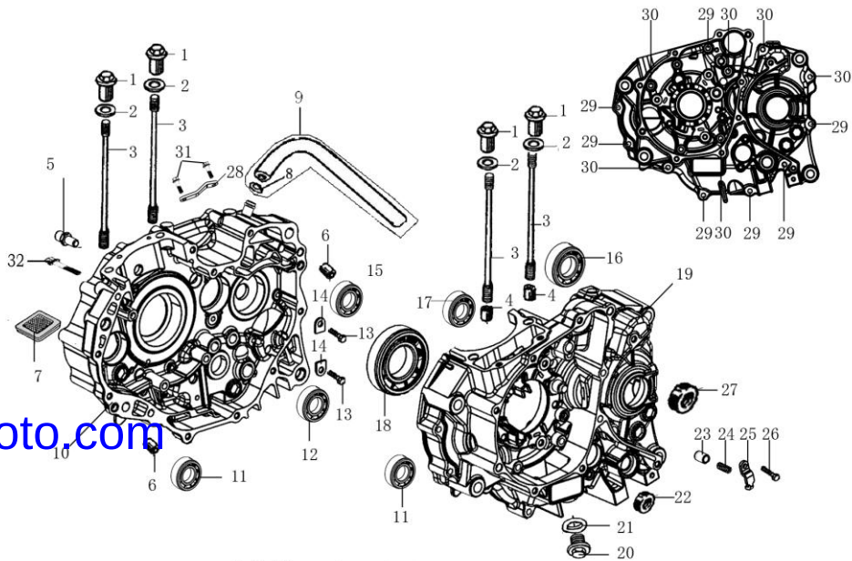
曲轴箱 CRANKCASE
