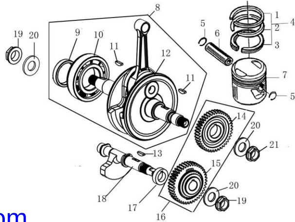
曲轴连杆部件 / 活塞 CRANKSHAFT CONNECTING-ROD ASSY/PISTON
