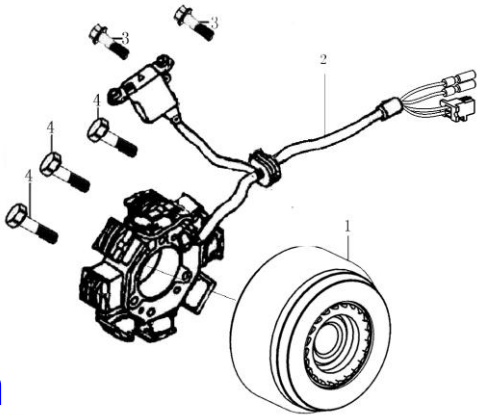
磁电机总成 MAGNETO COMP
