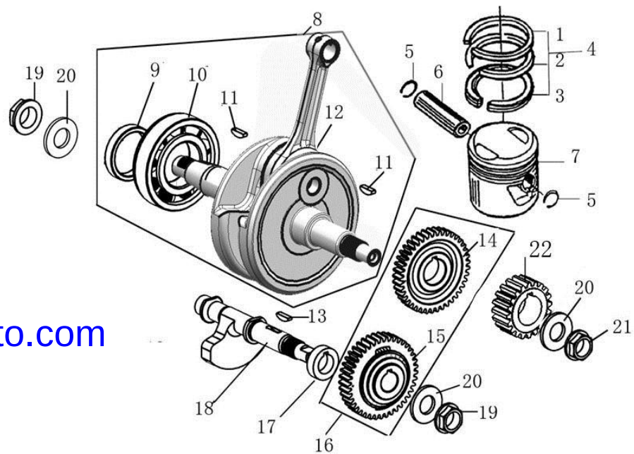
曲轴连杆部件 / 活塞 CRANKSHAFT CONNECTING-ROD ASSY/PISTON
