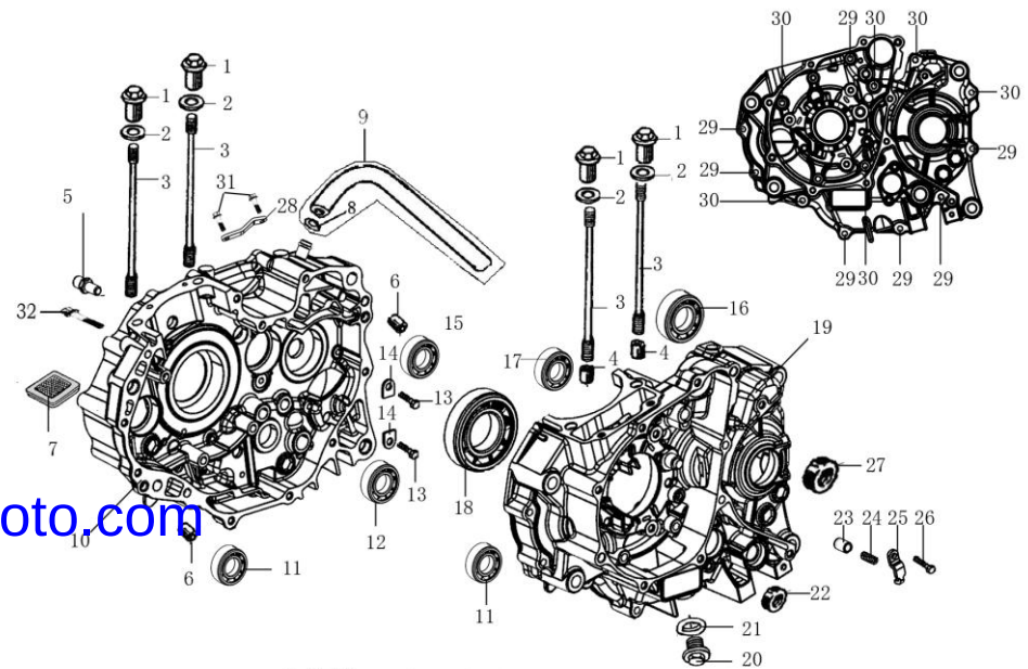
曲轴箱 CRANKCASE
