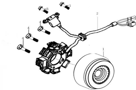
磁电机总成 MAGNETO COMP
