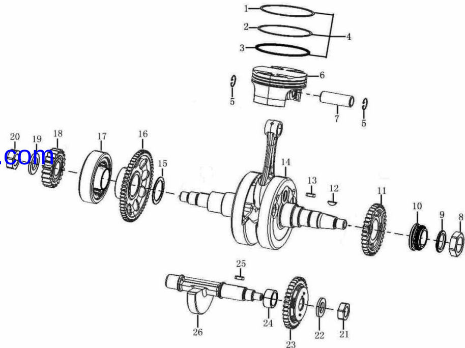
曲轴连杆部件 / 活塞 CRANKSHAFT CONNECTING-ROD ASSY/PISTON
