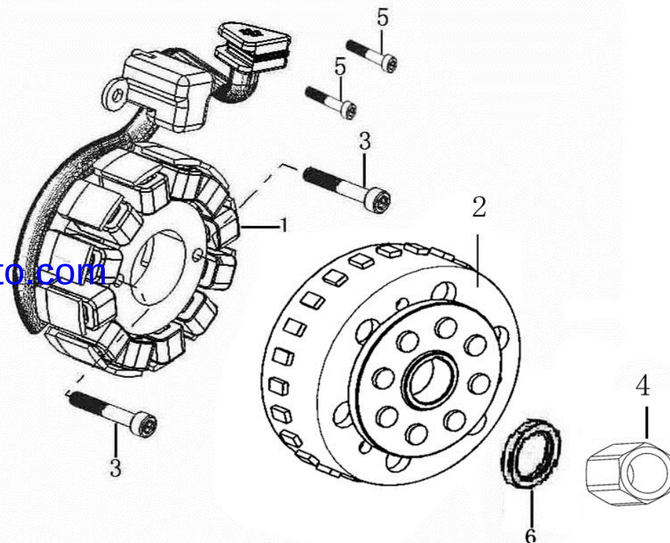
磁电机总成 MAGNETO COMP
