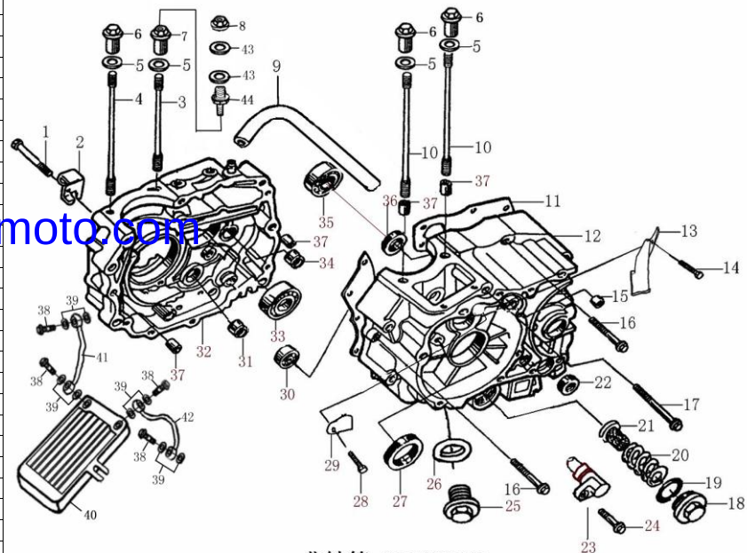
曲轴箱 CRANKCASE
