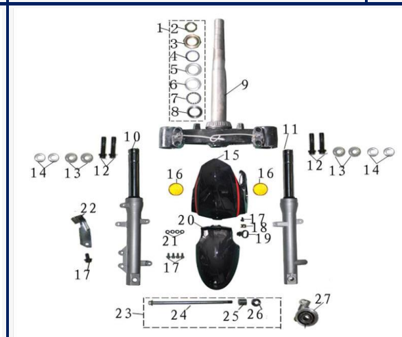
FIGURA N°12: TENEDOR Y BARRAS
