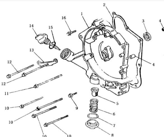
FIGURA N°23: COBERTOR COMPLETO RH
