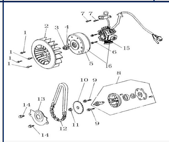
FIGURA N°30: GENERADOR Y BOMBA DE ACEITE
