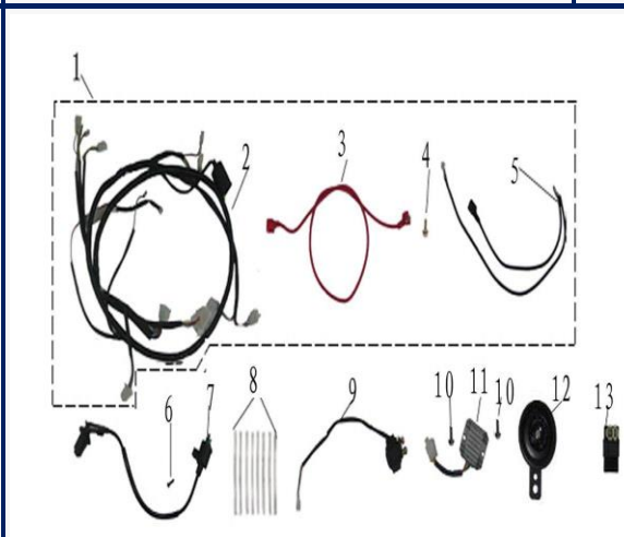
FIGURA N°11: SISTEMA ELECTICO
