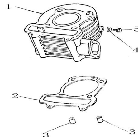
FIGURA N°24: CILINDRO
