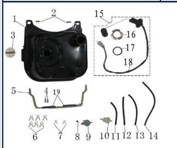
FIGURA N°10: TANQUE DE GASOLINA
