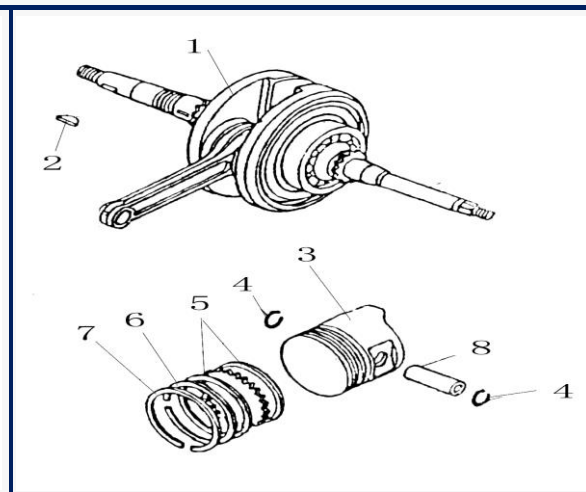
FIGURA N°27: CIGÜEÑAL Y PISTON
