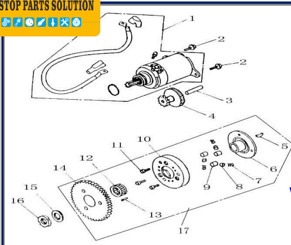
FIGURA N°37: ESTATER
