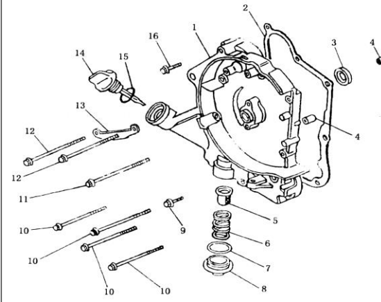
FIGURA N°35: CARTER RH
