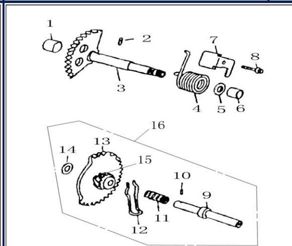
FIGURA N°41: EJE DE RATCH
