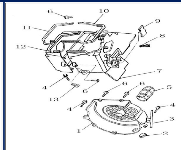
FIGURA N°42: CONDUCTOR DE ENFRIAMIENTO
