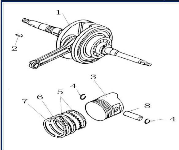
FIGURA N°40: PISTON Y CIGÜEÑAL
