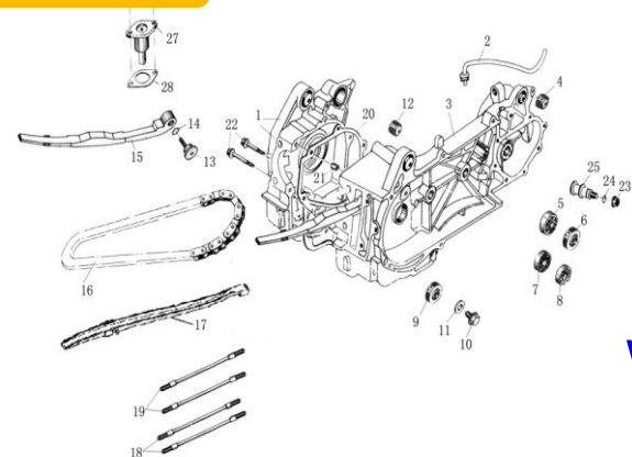
FIGURA N°31: CARTER DE MOTOR
