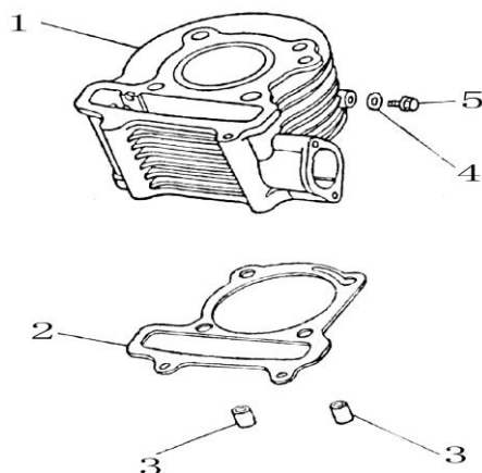
FIGURA N°34: CILINDRO
