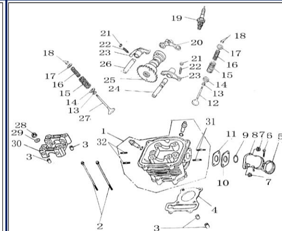
FIGURA N°33: CULATA
