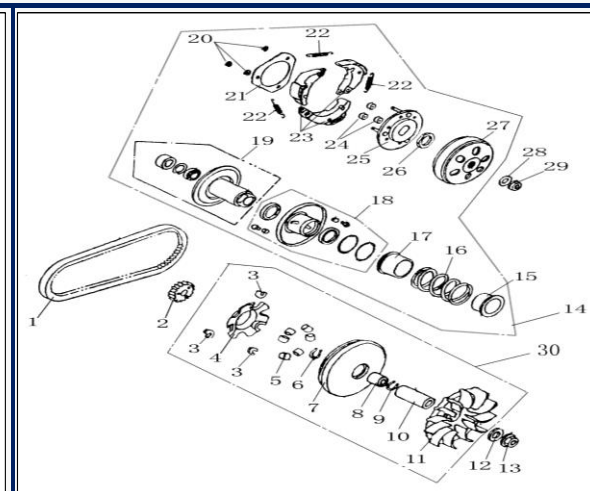
FIGURA N°39: CLUTCH
