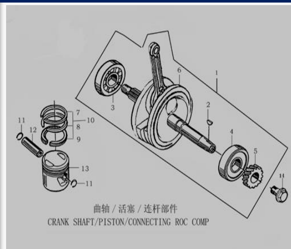
FIGURA N°22: CIGÜEÑAL
