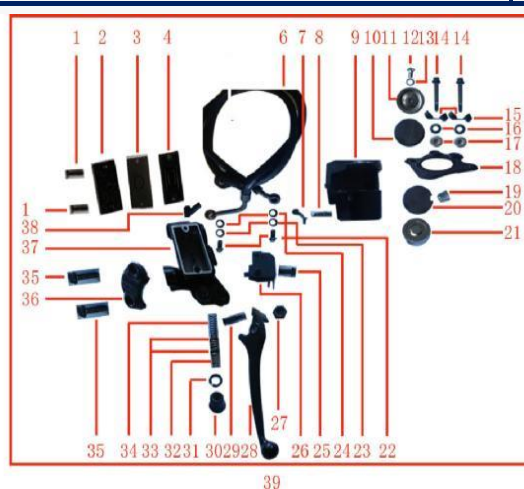
FIGURA N°11: FRENO DELANTERO
