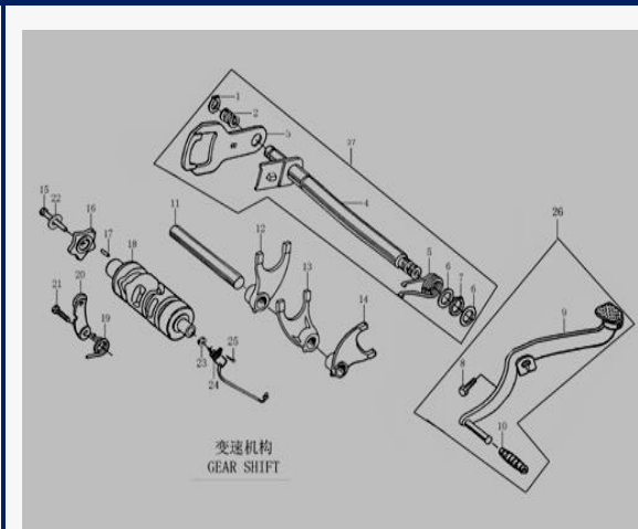
FIGURA N°24: MECANISMO DE CAMBIOS
