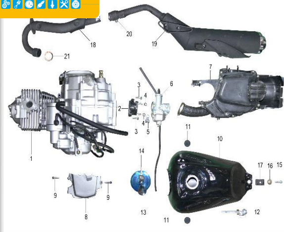
FIGURA N°1: ESCAPE, TANQUE, FILTRO Y MOTOR
