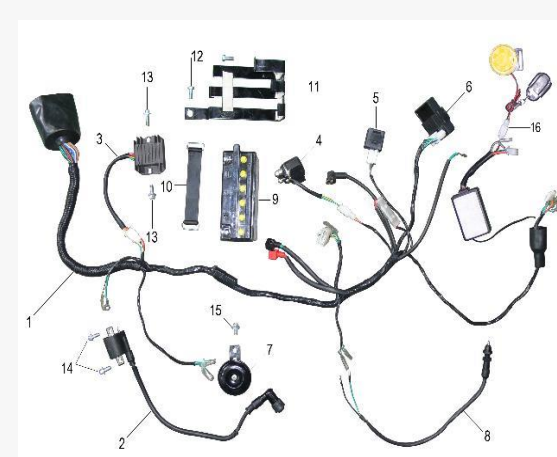
FIGURA N°3: SISTEMA ELECTRICO
