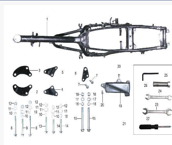
FIGURA N°15: CHASIS
