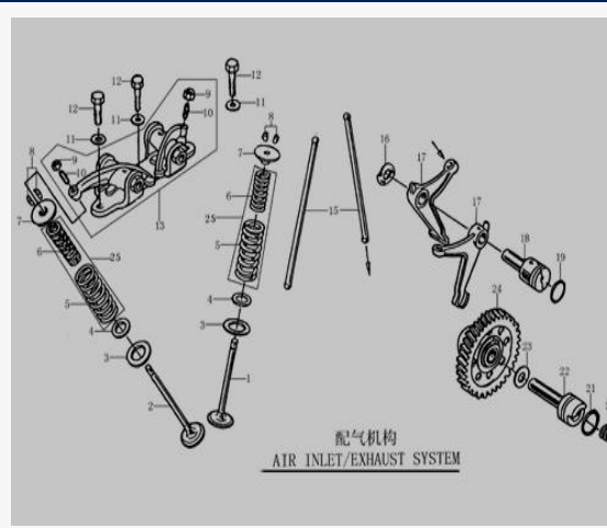
FIGURA N°17: VALVULAS
