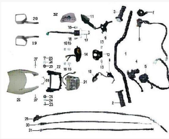
FIGURA N°5: TIMON
