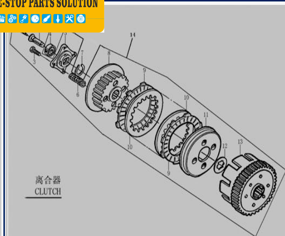
FIGURA N°19: CLUTCH
