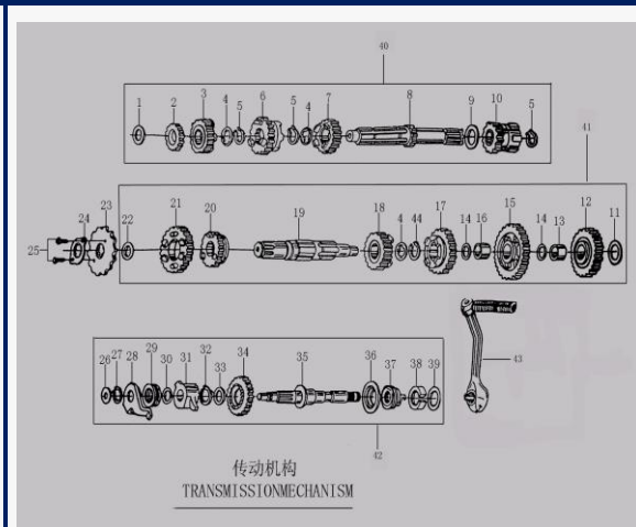
FIGURA N°23: MECANISMO DE TRANSMISION
