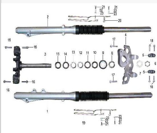
FIGURA N°4: TREN DELANTERO
