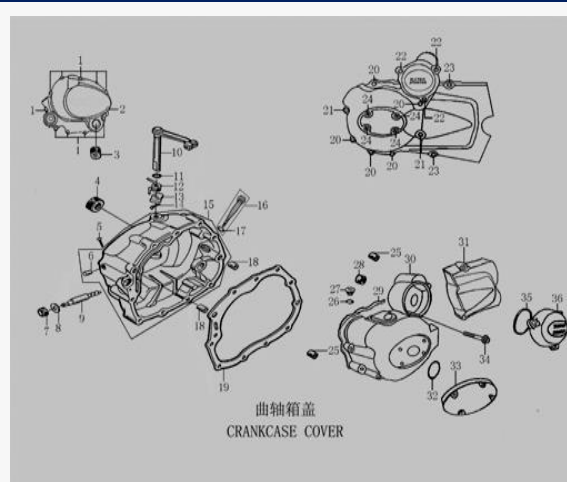
FIGURA N°18: CARTER RH
