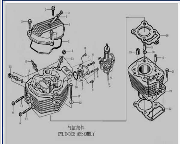
FIGURA N°16: CULATA
