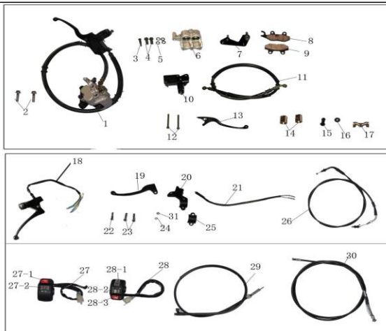
Figura N° 17: Sistema de control
