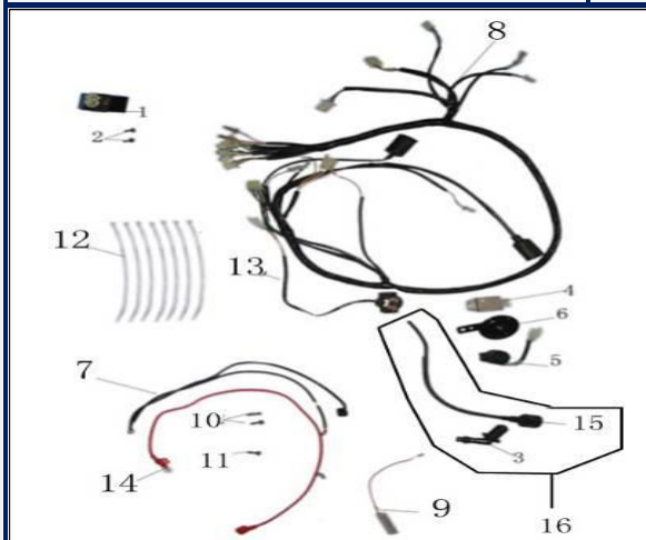
Figura N° 40: Harnes
