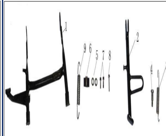
Figura N° 18: Patas
