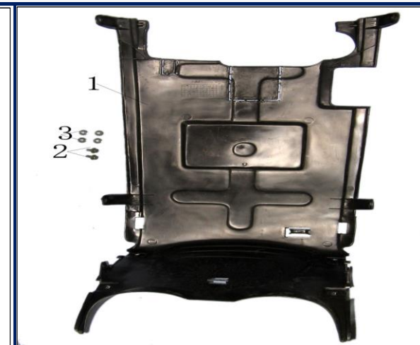
Figura N° 39: Cobertor de piso
