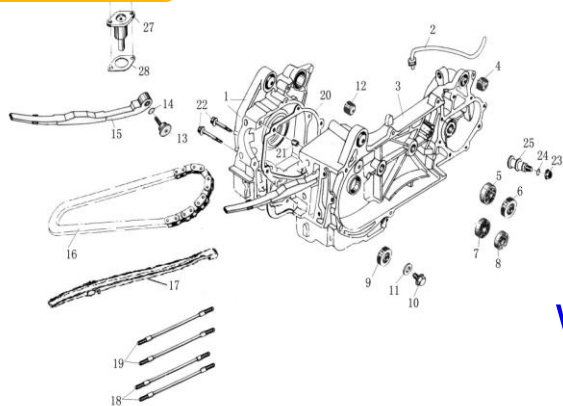
Figura N° 1: Carter
