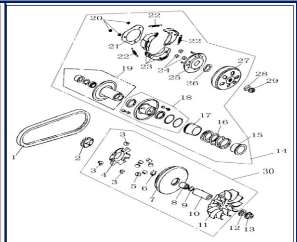
Figura N° 9: Clutch
