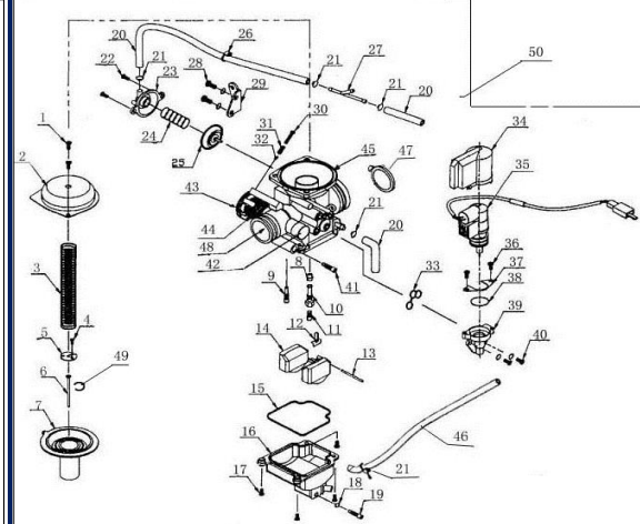
Figura N° 15: Carburador
