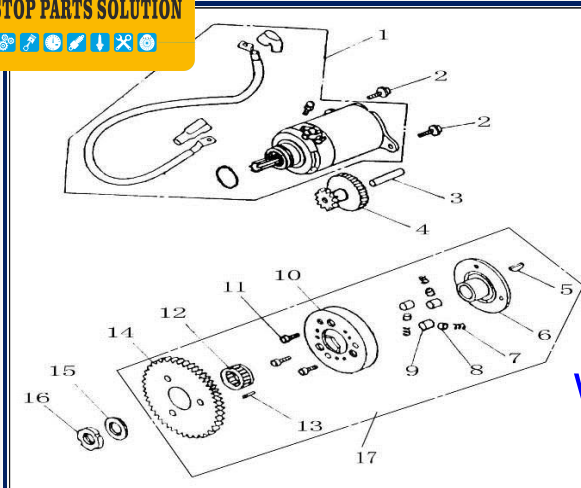
Figura N° 7: Estarter
