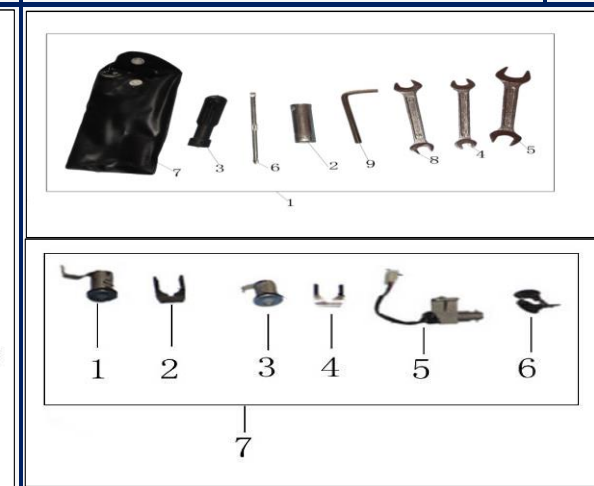
Figura N° 42: Kit de herramienta y kit de registro
