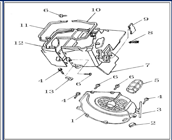
Figura N° 12: Conducto de enfriamiento
