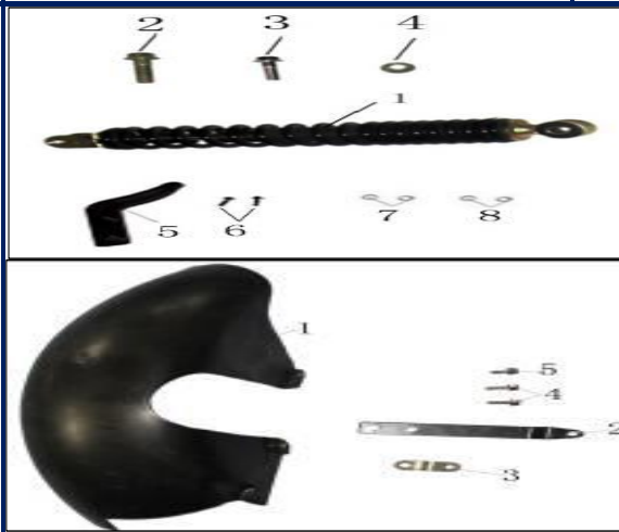
Figura N° 35: Amortiguador y salpicadera
