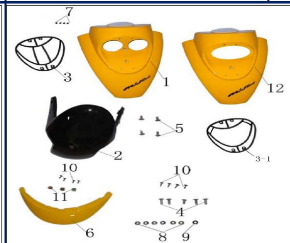
Figura N° 30: Cobertor frontal
