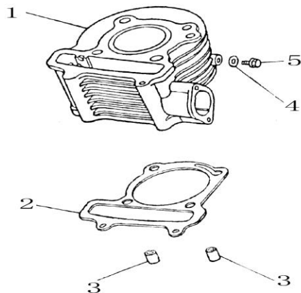
Figura N° 4: Cilindro
