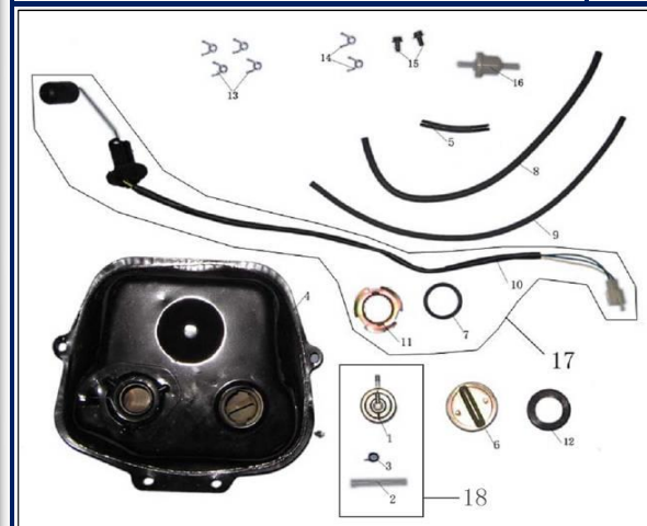
Figura N° 22: Tanque de gasolina
