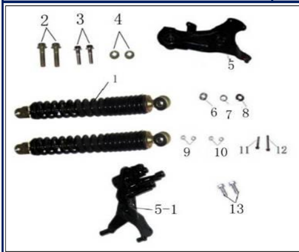
Figura N° 34: Amortiguador
