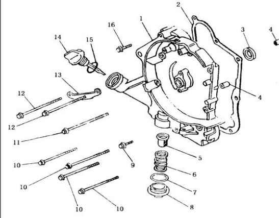
Figura N° 5: Carter
