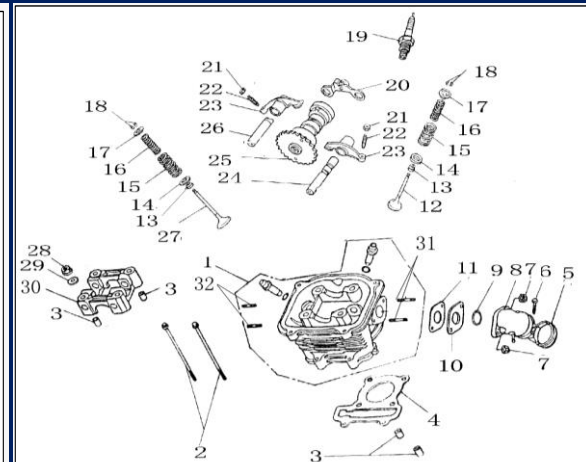
Figura N° 3: Culata
