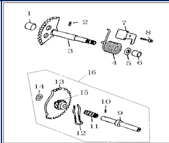
Figura N° 11: Eje de ratch
