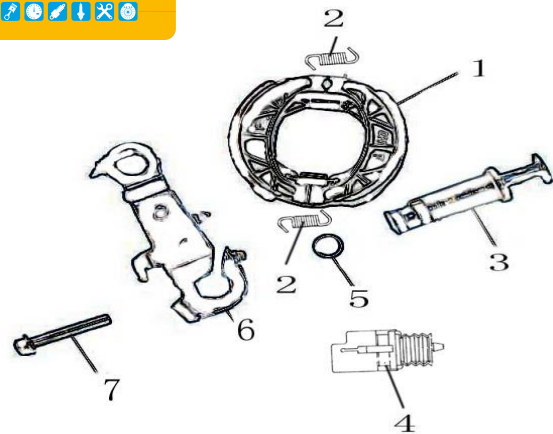
Figura N° 13: Fricciones
