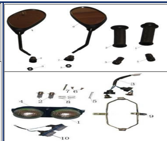
Figura N° 27: Retrovisores y silvin
