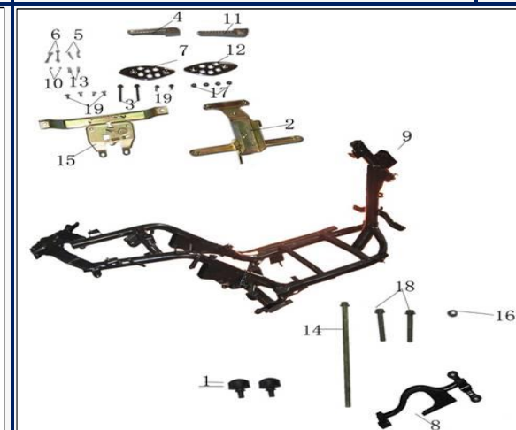
Figura N° 41: Chasis
