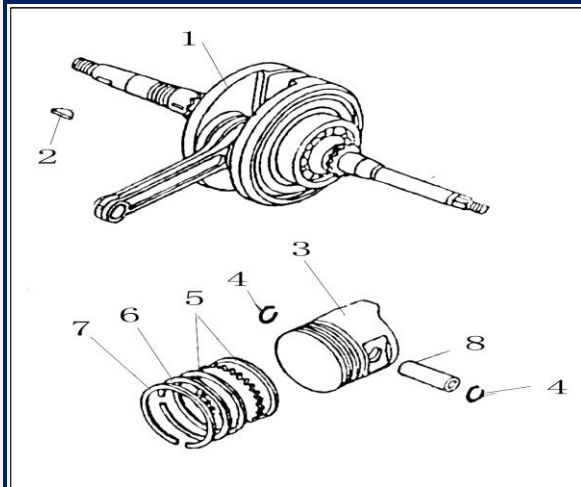
Figura N° 10: Pisotn y cigüeñal
