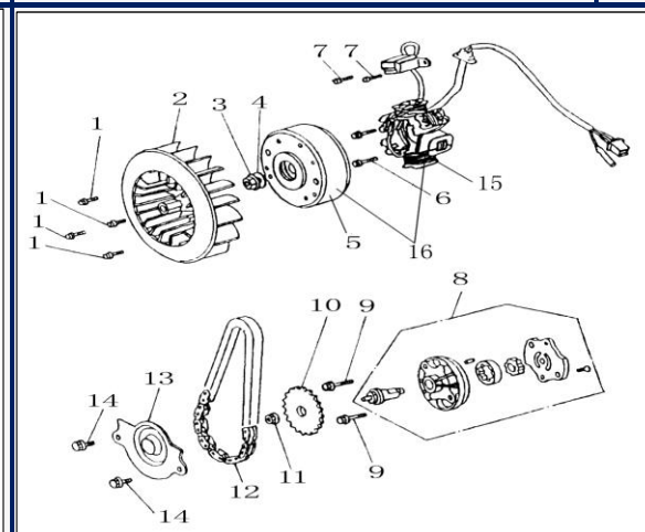
Figura N° 6: Planta y bomba de aceite
