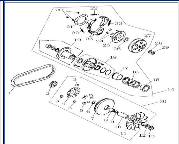
Figura N° 9: Clutch
