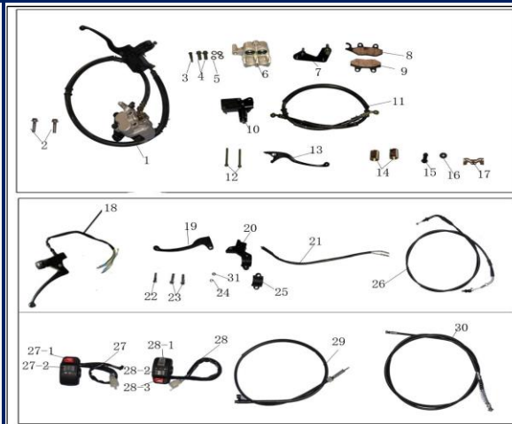
Figura N° 17: Sistema de control
