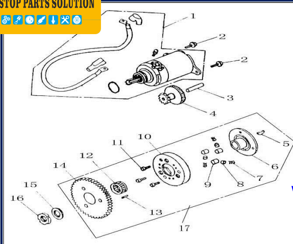
Figura N° 7: Starter
