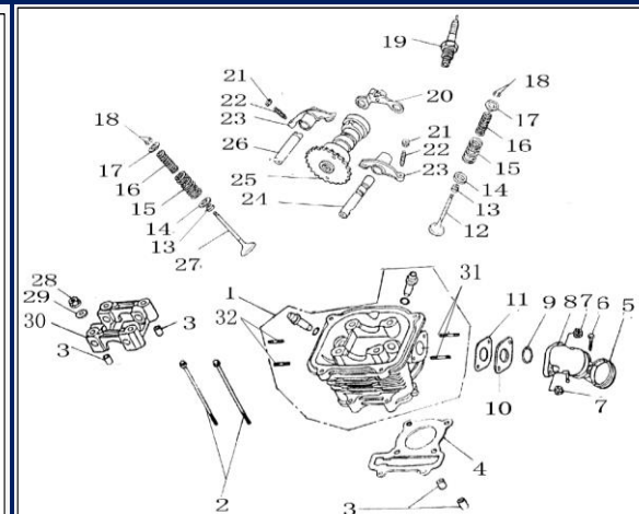
Figura N° 3: Culata
