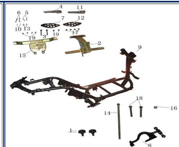
Figura N° 39: Chasis
