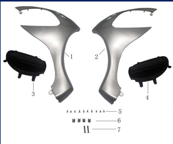
Figura N° 30: Protector delantero
