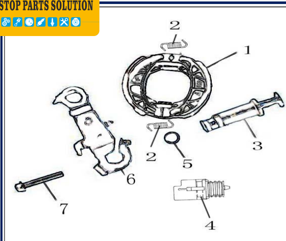
Figura N° 13: Fricciones
