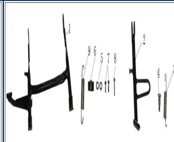
Figura N° 18: Patas
