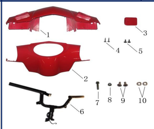
Figura N° 36: Timon
