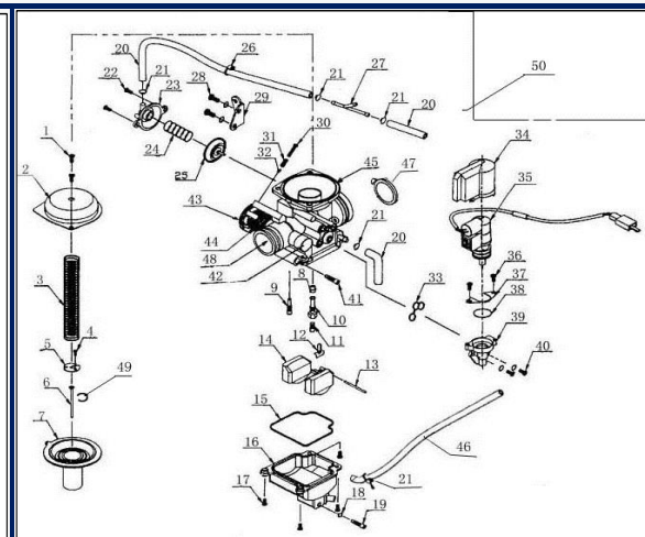
Figura N° 15: Carburador
