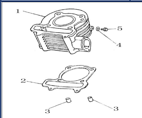
Figura N° 4: Cilindro
