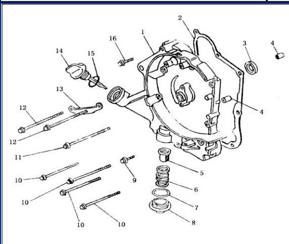
Figura N° 5: Carter
