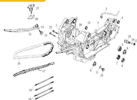
Figura N° 1: Carter
