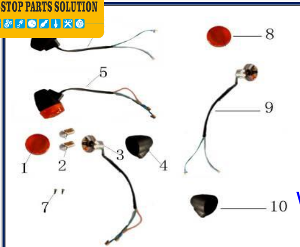
Figura N° 19: Pidevias
