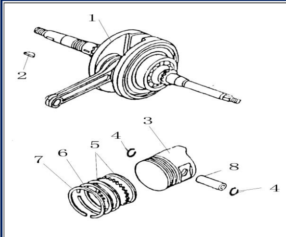
Figura N° 10: Piston y cigüeñal
