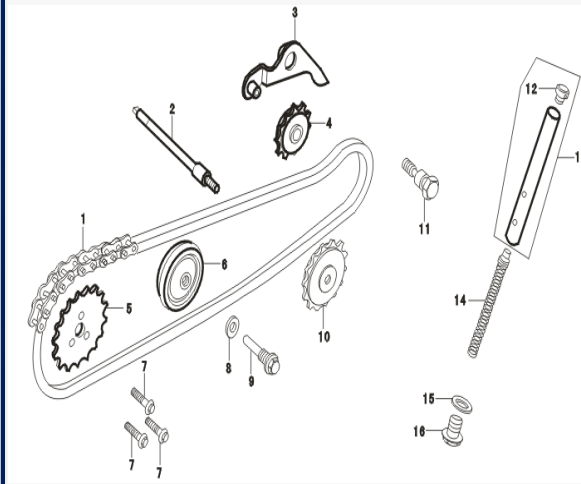
FIGURA N°16: CADENA DE TIEMPO
