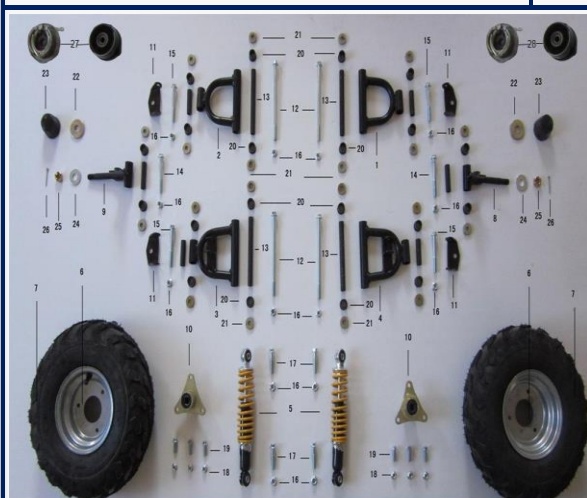
FIGURA N°4: DIRECCION DELANTERA COMPLETA
