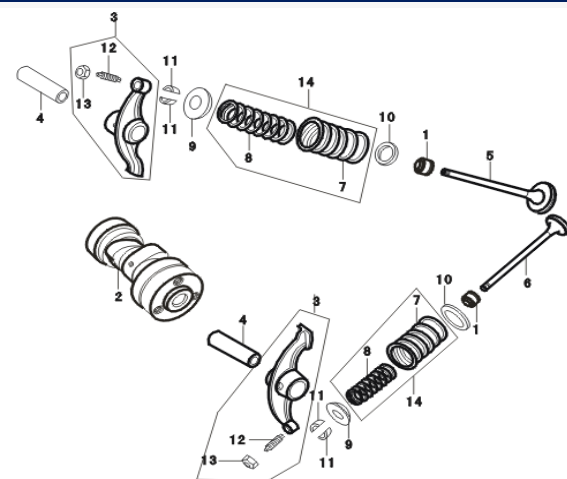
FIGURA N°9: EJE DE LEVAS, BALANCIN Y VALVULAS
