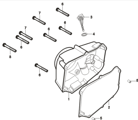
FIGURA N°10: TAPADERA DE CARTER RH
