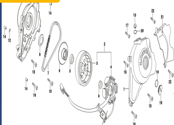
FIGURA N°13: TAPADERA DE VOLANTE
