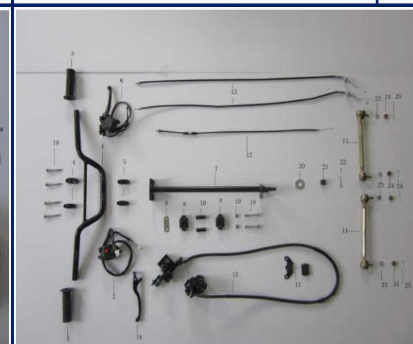
FIGURA N°6: TIMON COMPLETO
