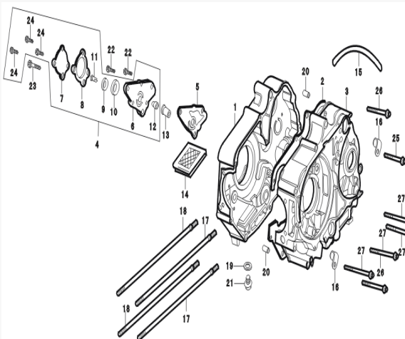
FIGURA N°11: CARTER COMPLETO
