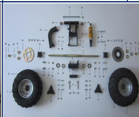
FIGURA N°5: MULETA TRASERA COMPLETA
