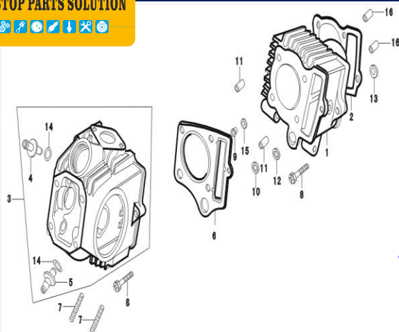
FIGURA N°7: CILINDRO Y CULATA
