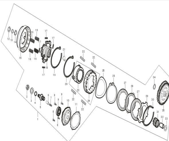
FIGURA N°12: CANASTA DE CLUTCH
