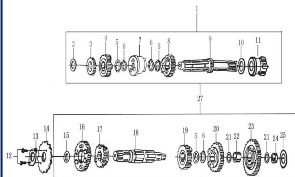
主副轴组合 TRANSMISSION MAIN, COUNTER SHAFT
