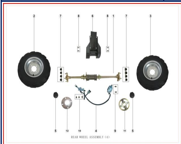
FIGURA N°4: FRENO LLANTAS Y PUENTE TRASERO
