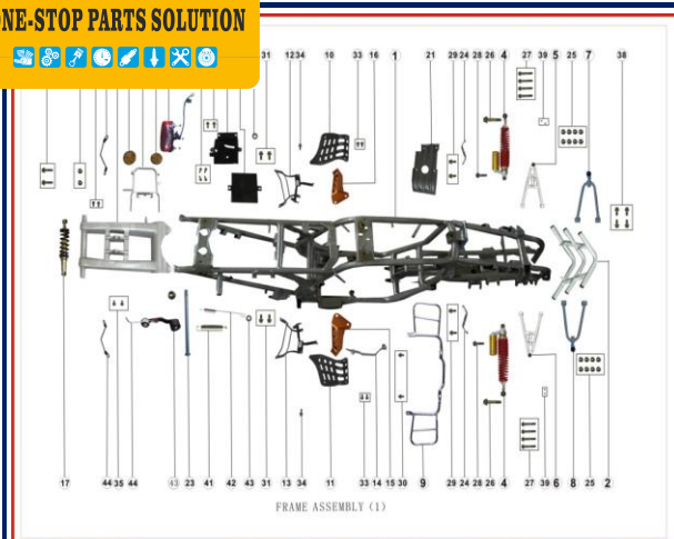
FIGURA N°1: CHASIS
