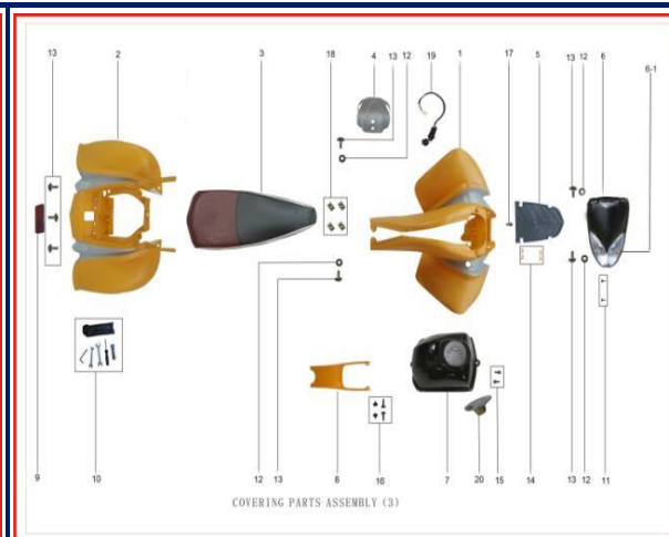
FIGURA N°3: CARROCERIA
