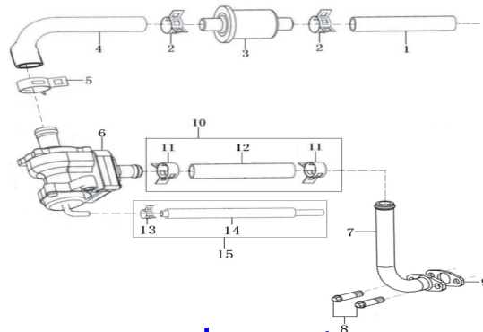
废气再循环系统 EXHAUST GAS RECIRCULATION SYSTEM
