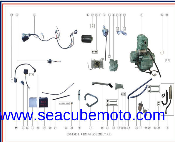
FIGURA N°2: MOTOR
