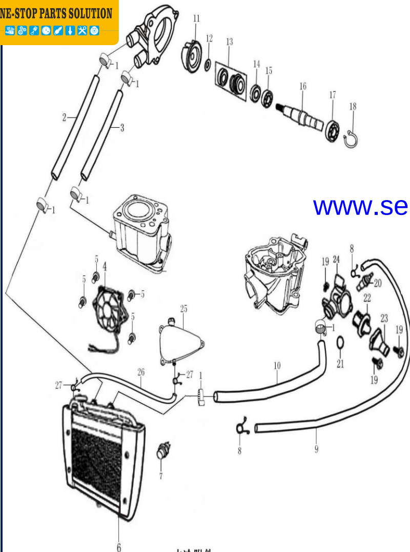
水冷附件 WATER COOLING SYSTEM
