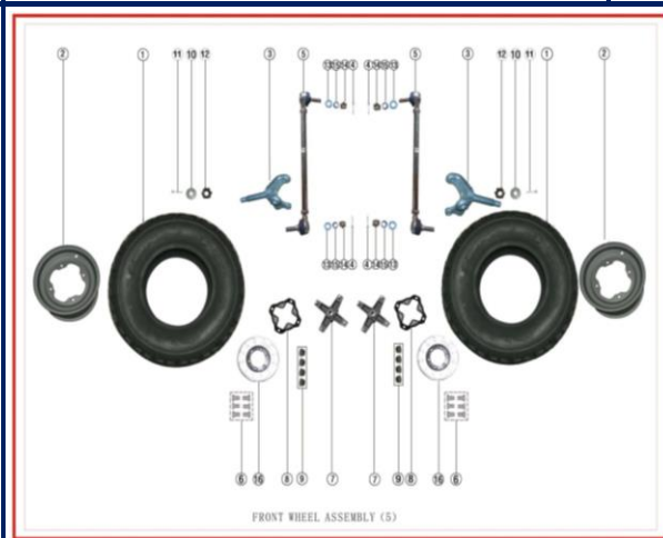
FIGURA N°5: DIRECCION, LLANTA DELANTERA
