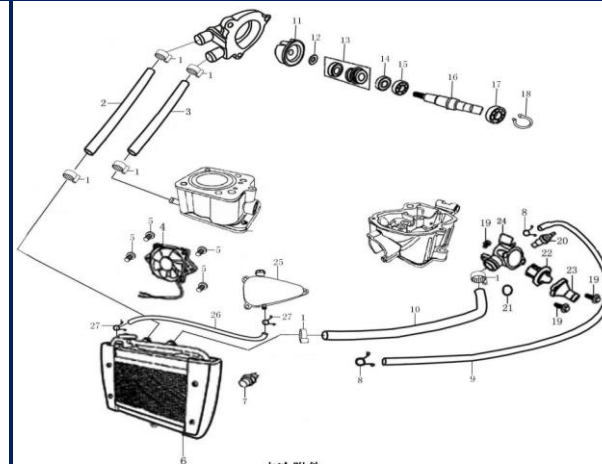
水冷附件 WATER COOLING SYSTEM
