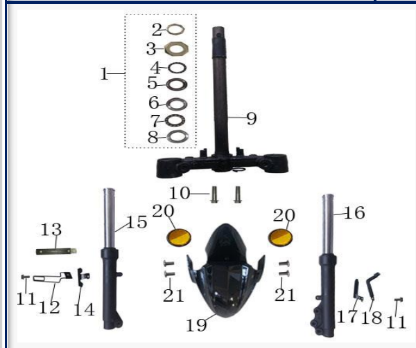
FIGURA N°22: TREN DELANTERO
