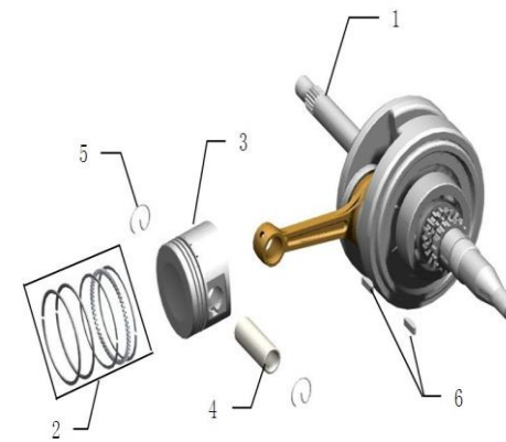
FIGURA N°15: CIGÜEÑAL
