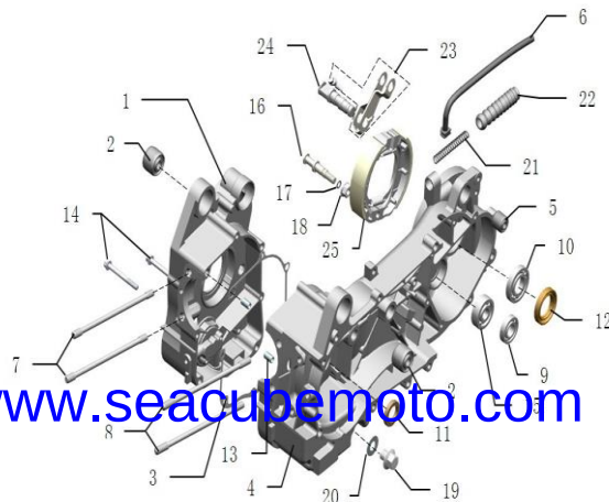
FIGURA N°14: CARTER RH
