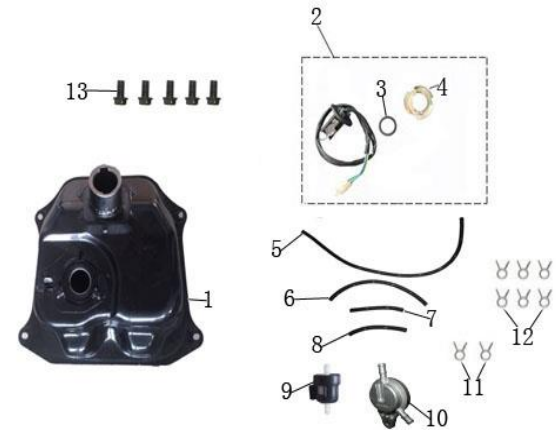
FIGURA N°27: TANQUE DE GASOLINA
