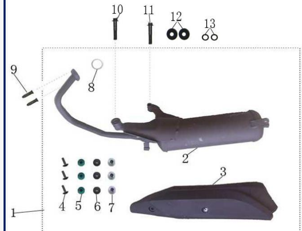
FIGURA N°30: ESCAPE
