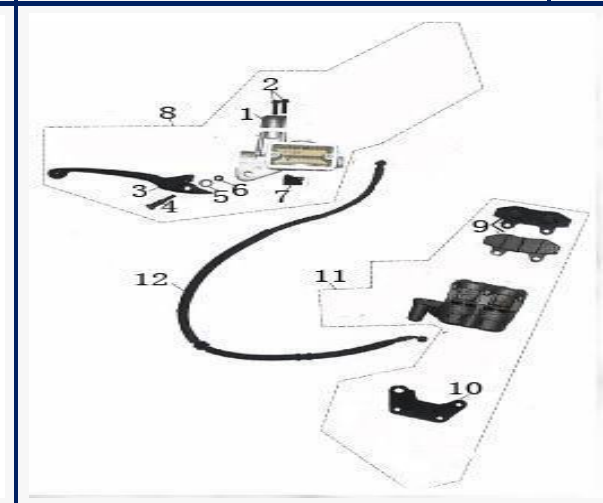
FIGURA N°24: FRENO HIDRÁULICO DELANTERO
