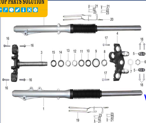
Figura N° 13: Barras y T de barras
