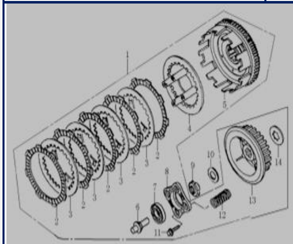
Figura N° 4: Clutch
