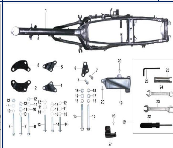
Figura N° 12: Chasis
