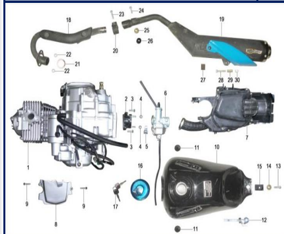
Figura N° 22: Sistema de escape y tanque de gasolina
