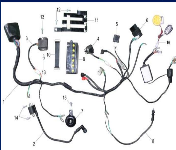
Figura N° 23: Harnes
