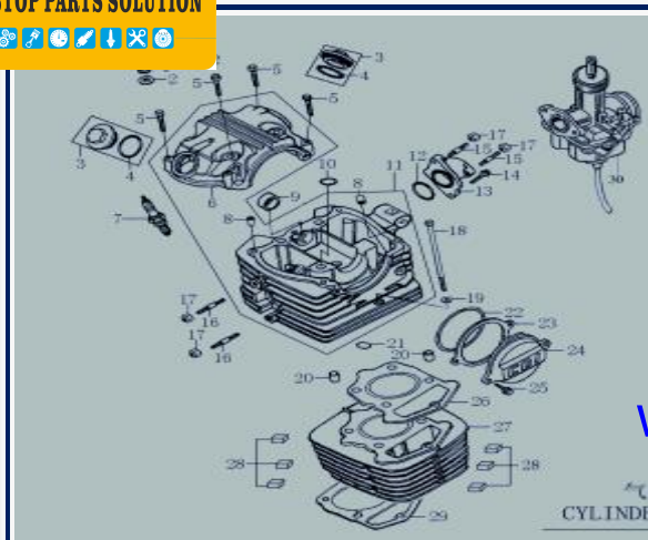
Figura N° 1: Motor
