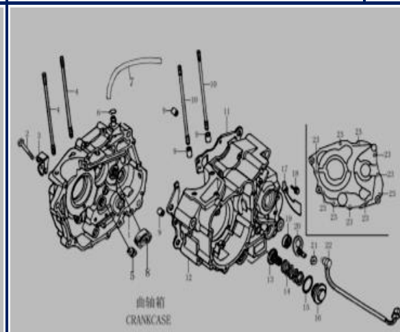
Figura N° 6: Carter
