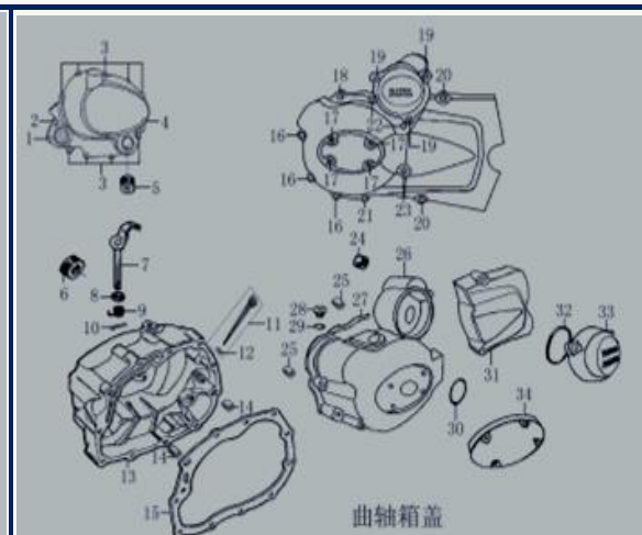
Figura N° 3: Tapadera de carter
