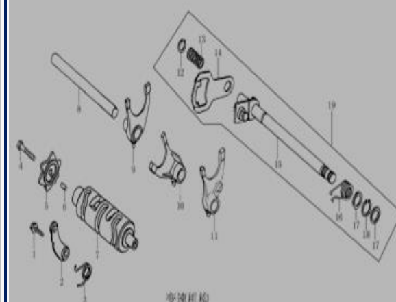
Figura N° 9: Mecanismo de cambios
