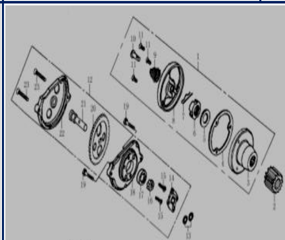
Figura N° 5: Bomba de aceite y filtro de centrifugo
