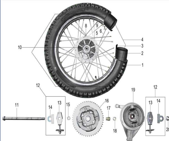
Figura N° 16: Llanta trasera
