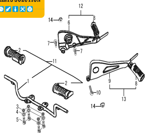
Figura N° 31: Reposapiés
