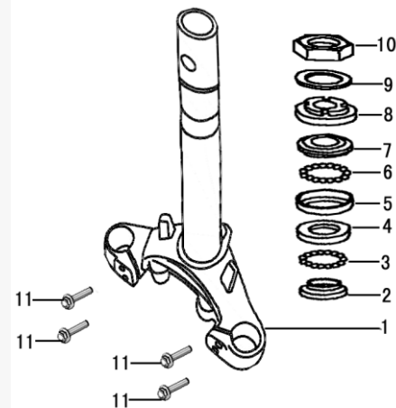
Figura N° 18: T de barras
