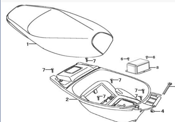
Figura N° 24: Sillón
