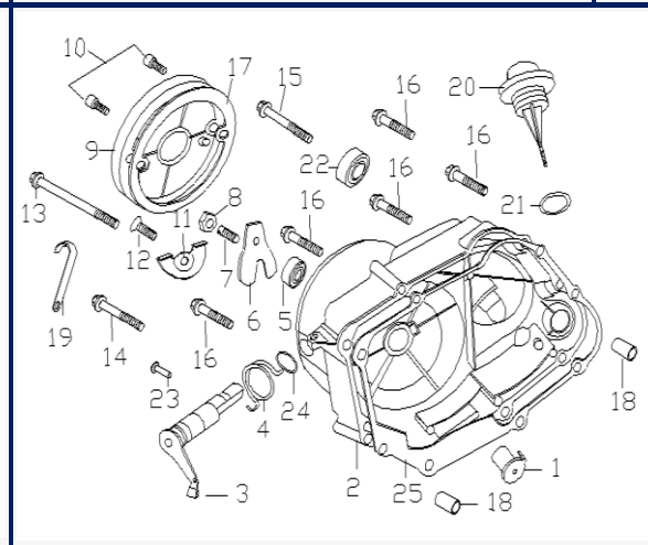
Figura N° 5: Tapadera de clutch
