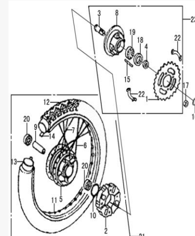
Figura N° 21: Llanta trasera
