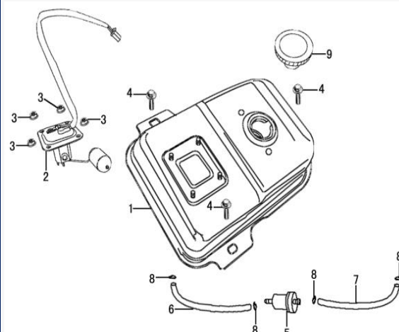
Figura N° 23: Tanque de gasolina
