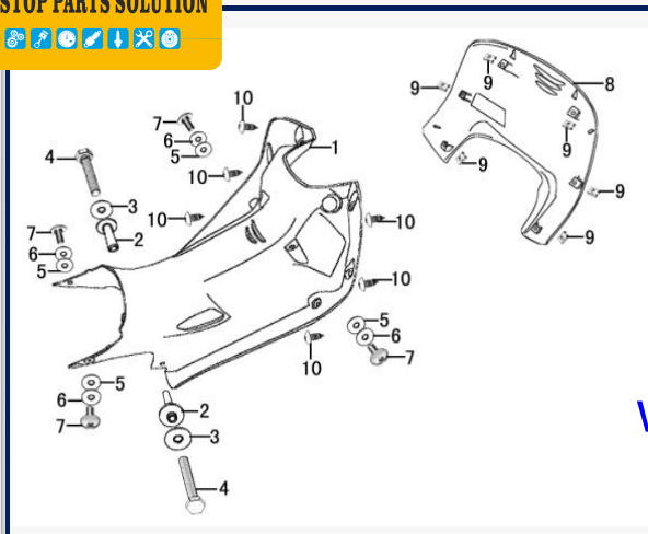
Figura N° 25: Cobertores
