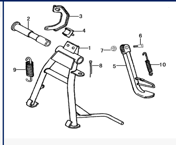
Figura N° 30: Pata lateral/doble
