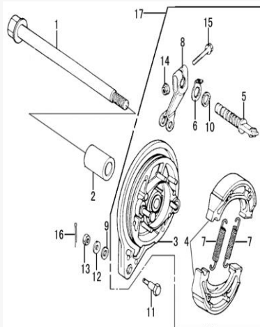
Figura N° 22: Freno trasero
