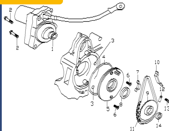
Figura N° 13: Motor de arranque
