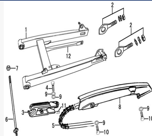
Figura N° 33: Muleta trasera
