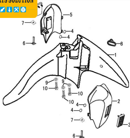
Figura N° 19: Lodera delantera
