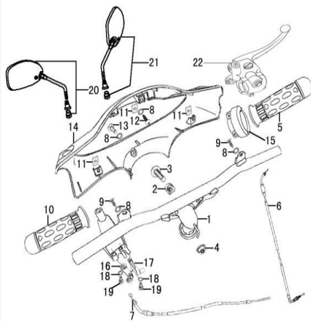
Figura N° 16: Timon
