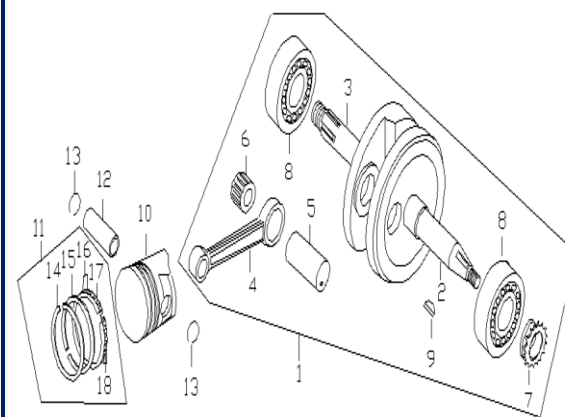
Figura N° 9: Cigüeñal
