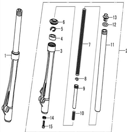
Figura N° 17: Barras
