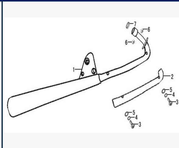
Figura N° 29: Escape
