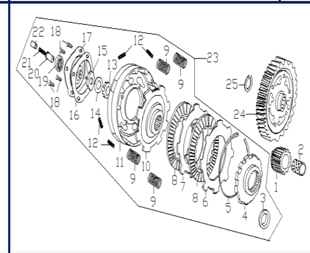
Figura N° 6: Clutch
