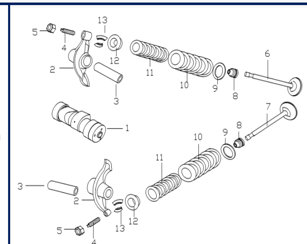
Figura N° 3: Valvulas
