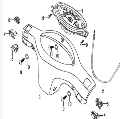
Figura N° 15: Tablero
