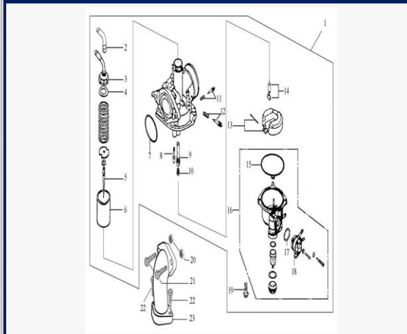
Figura N° 28: Carburador
