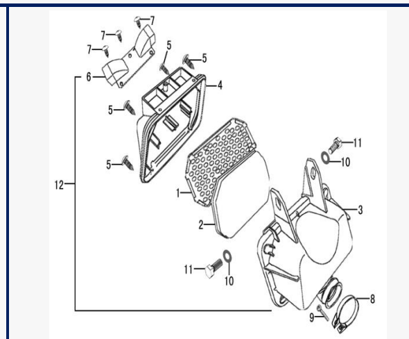
Figura N° 27: Filtro de aire
