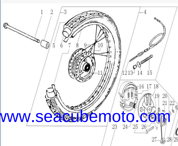
Figura N° 20: Llanta y freno delantero
