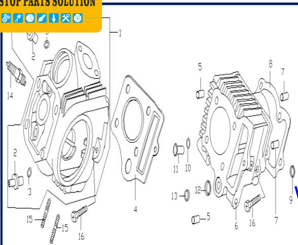
Figura N° 1: Culata
