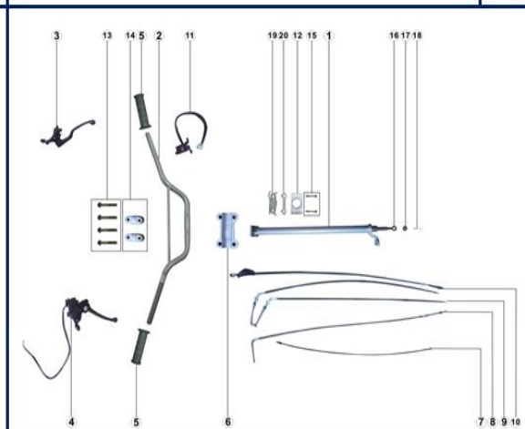
Figura N° 18: Controles
