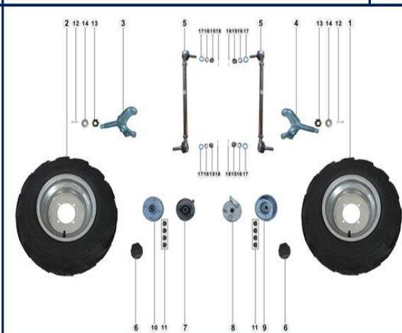
Figura N° 17: Tren delantero
