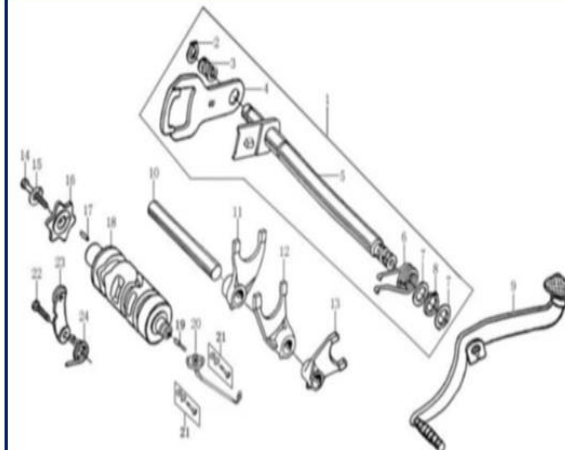
Figura N° 9: Mecanismo de cambios
