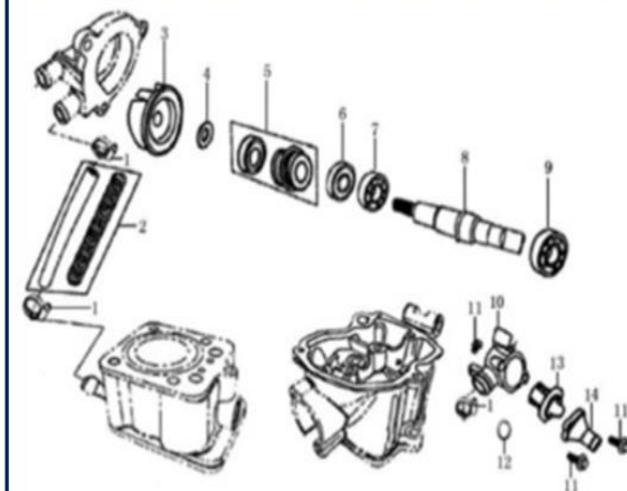
Figura N° 12: Sistema de enfriamiento
