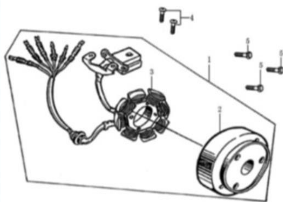
Figura N° 10: Magneto
