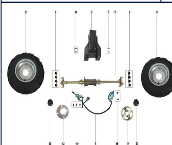
Figura N° 16: Eje trasero
