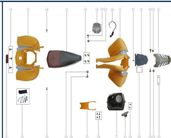
Figura N° 15: Cobertores
