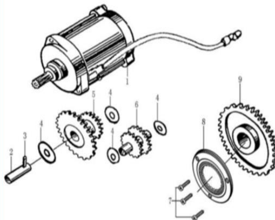
Figura N° 11: Estarter
