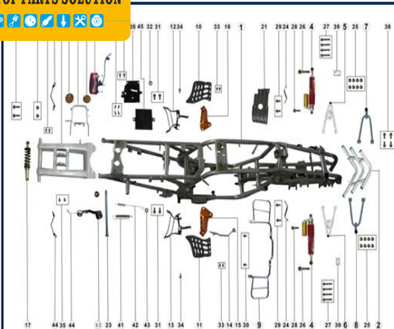
Figura N° 13: Chassis
