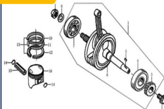
Figura N° 7: Cigüeñal y Piston
