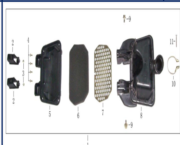
Figura N° 24: Filtro de aire
