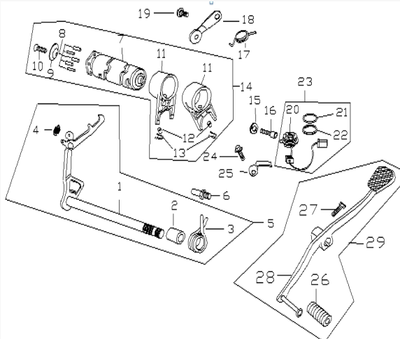
Figura N° 11: Pata de cambios
