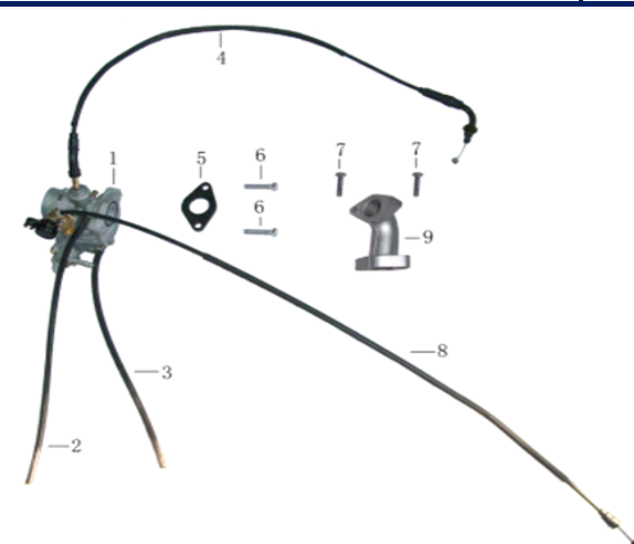
Figura N° 23: Carburador
