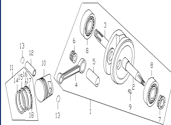
Figura N° 9: Cigüeñal
