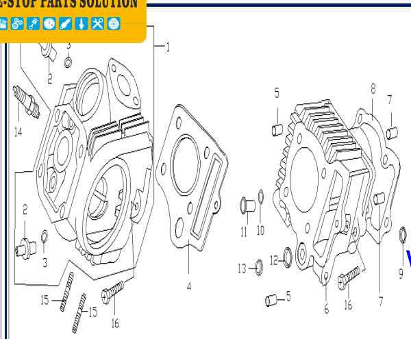
Figura N° 1: Culata
