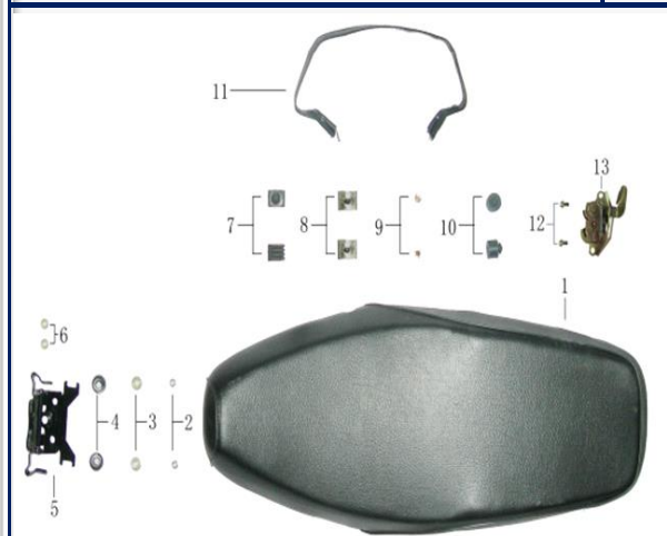
Figura N° 28: Sillon
