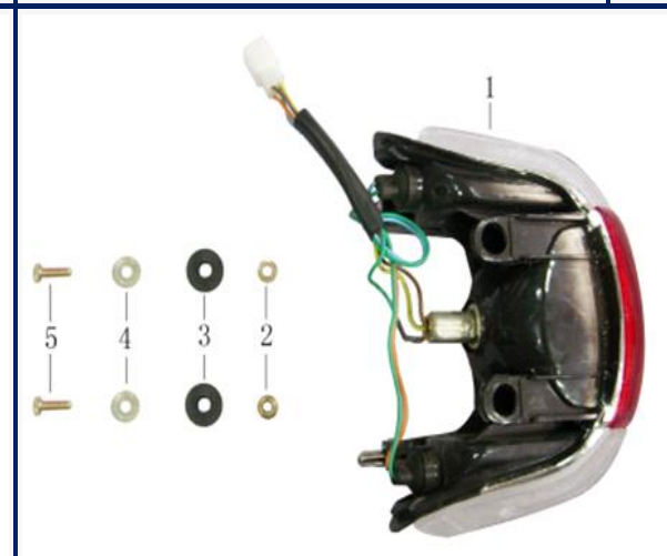
Figura N° 36: Stop
