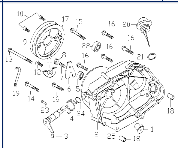
Figura N° 5: Tapadera de clutch
