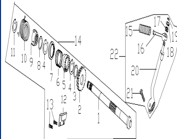
Figura N° 12: Mecanismo de arranque
