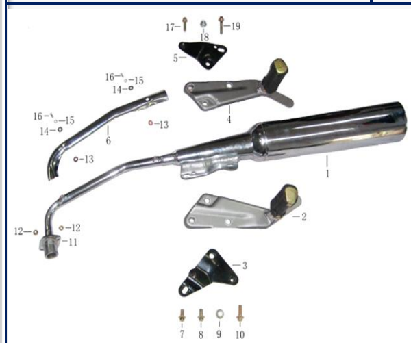
Figura N° 34: Escape
