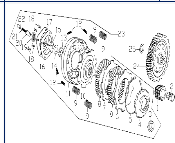
Figura N° 6: Clutch
