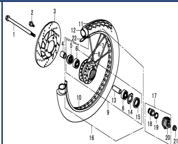
Figura N° 39: Llanta delantera
