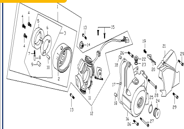
Figura N° 7: Kit de arranque
