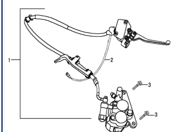
FIGURA N°42: FRENO DE DISCO DELANTERO
