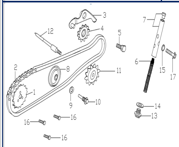
Figura N° 4: Kit de sprocket
