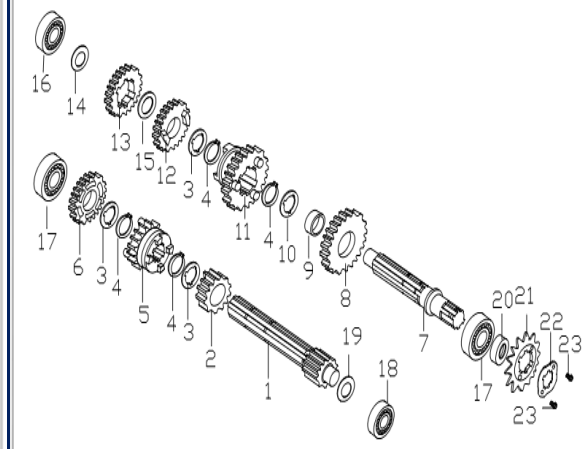
Figura N° 10: Transmision
