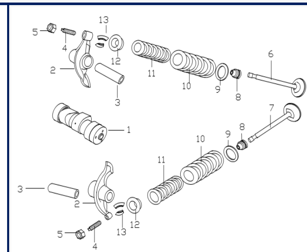
Figura N° 3: Valvulas
