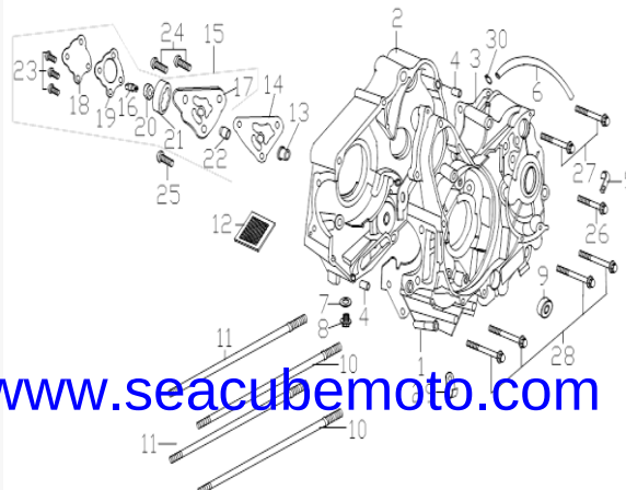
Figura N° 8: Carter
