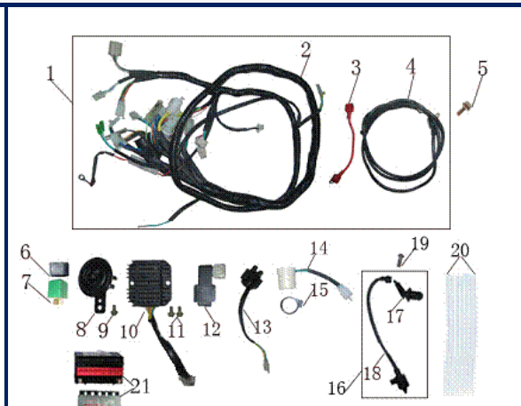
FIGURA N°9: SISTEMA ELECTRICO
