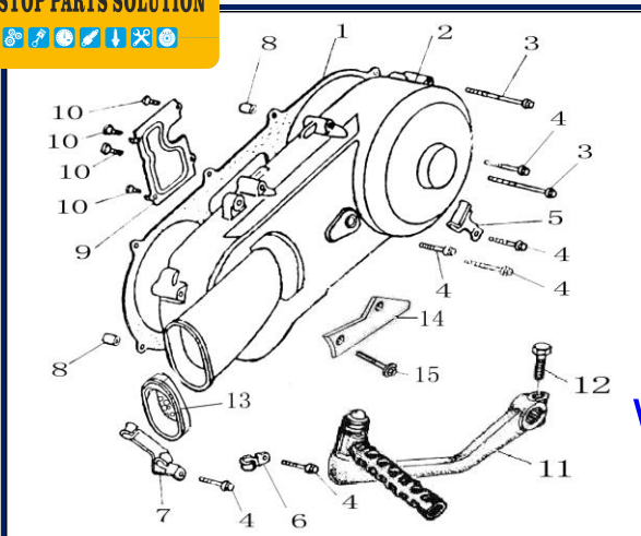
FIGURA N°25: TAPADERA DE CLUTCH
