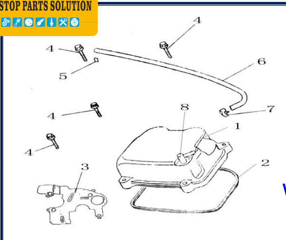
FIGURA N°19: TAPADERA DE CULATA
