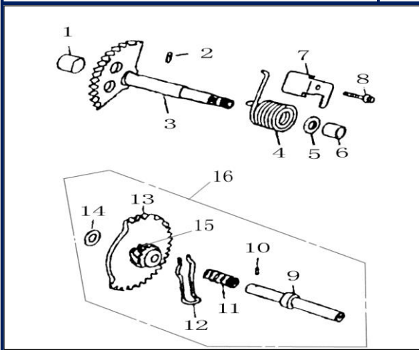
FIGURA N°28: EJE DE RATCH
