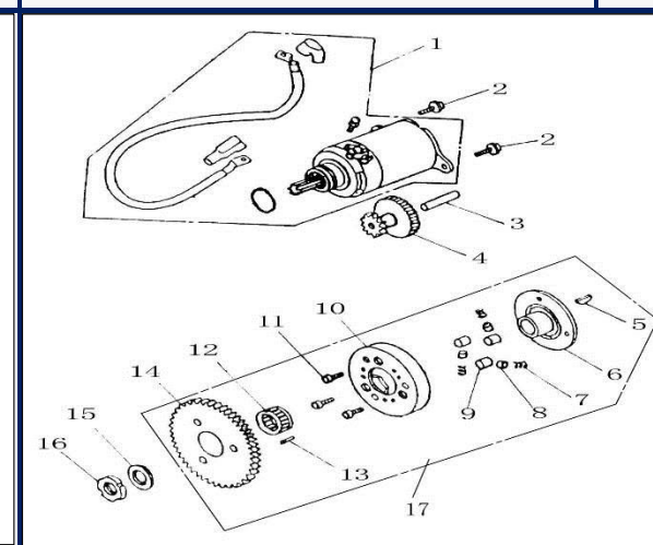
FIGURA N°24: ESTARTER
