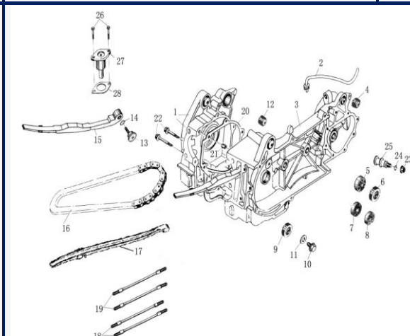
FIGURA N°18: CARTER DE MOTOR
