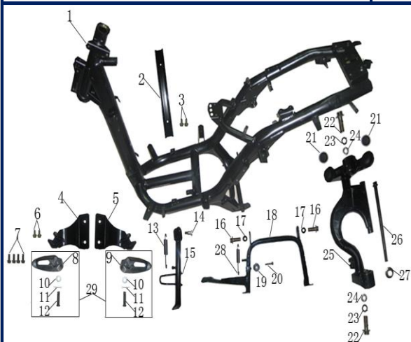
FIGURA N°16: CHASIS
