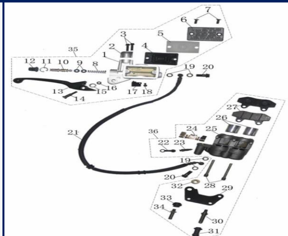
FIGURA N°12: BOMBA DE FRENO
