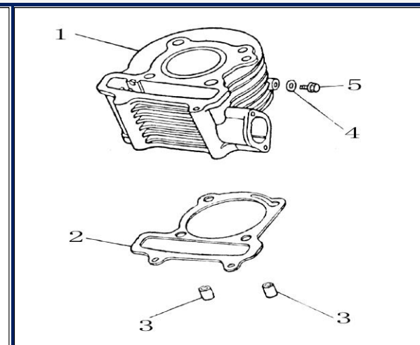
FIGURA N°21: CILINDRO
