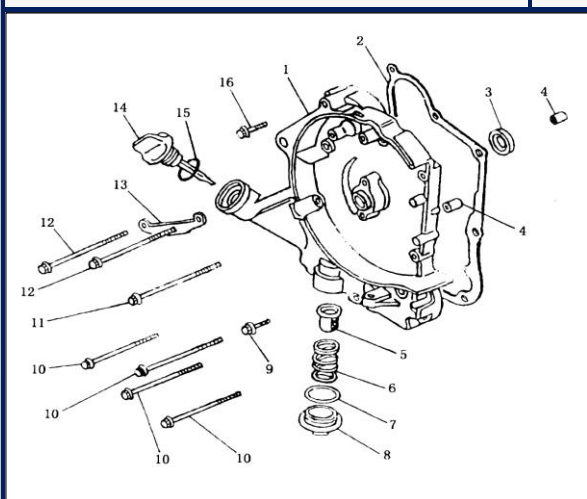
FIGURA N°22: CARTER RH
