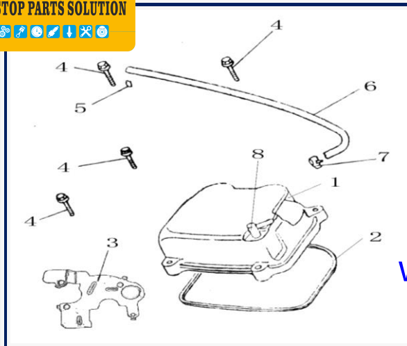
Figura N° 7: Tapadera de culata
