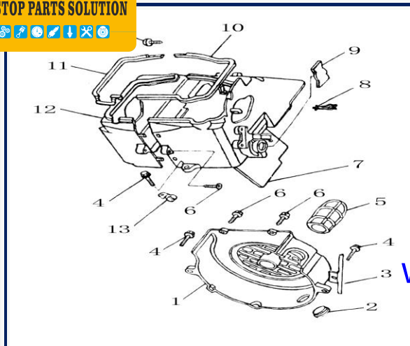
Figura N° 13: Conduto de enfriamiento
