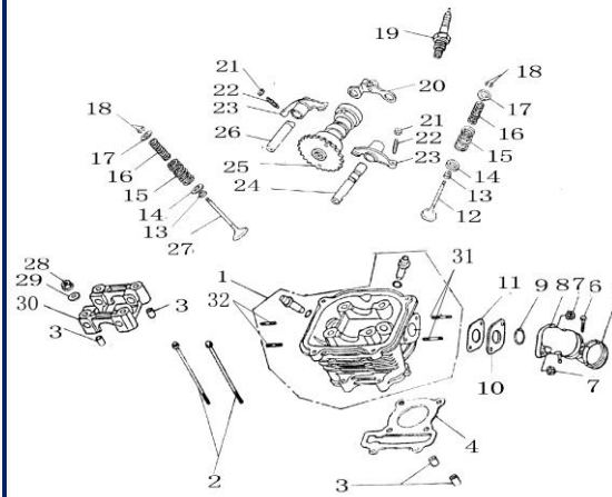
Figura N° 6: Culata
