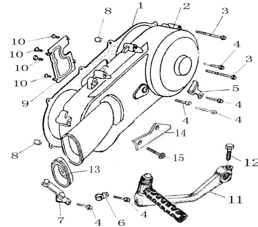
Figura N° 3: Embrague
