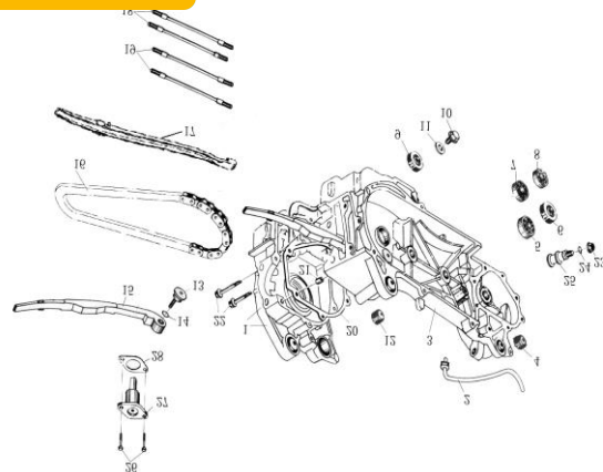
Figura N° 1: Motor
