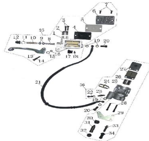
Figura N° 29: Sistema de frenos
