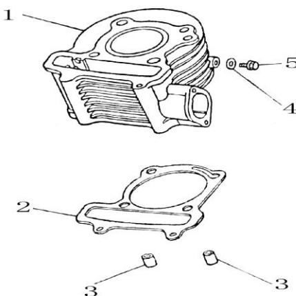
Figura N° 5: Cilindro
