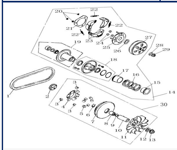
Figura N° 10: Cluth
