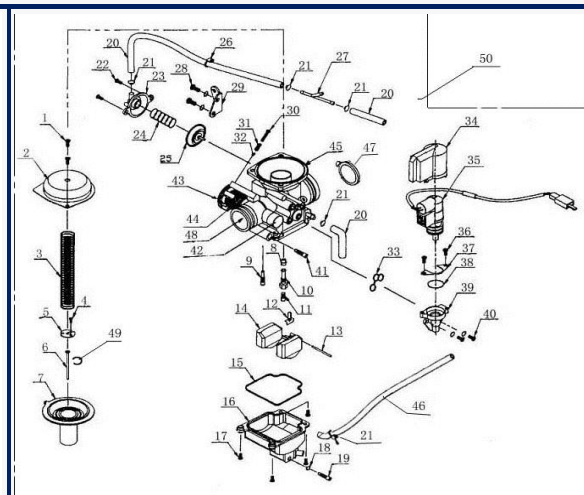
Figura N° 15: Carburador
