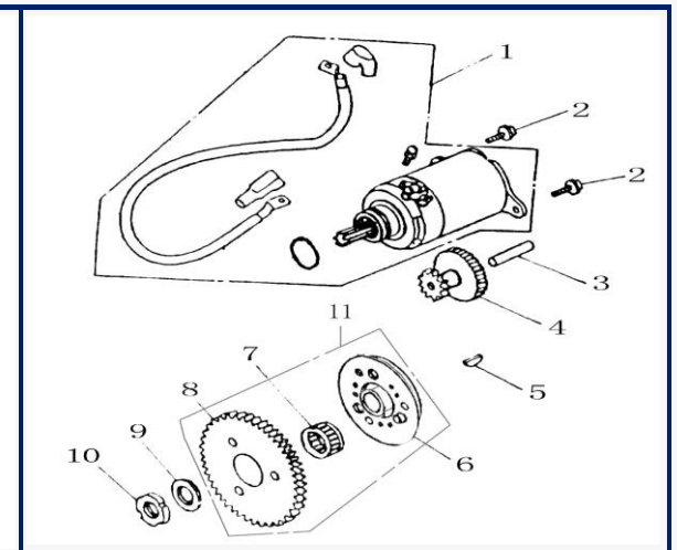
Figura N° 9: Estarter
