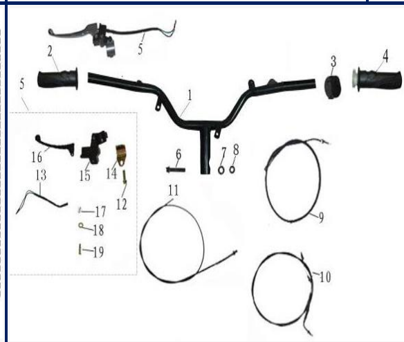
Figura N° 18: Timon
