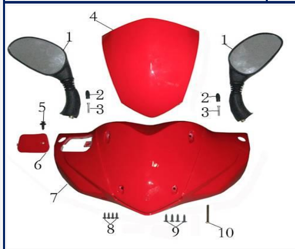
Figura N° 16: Cobertor frontal
