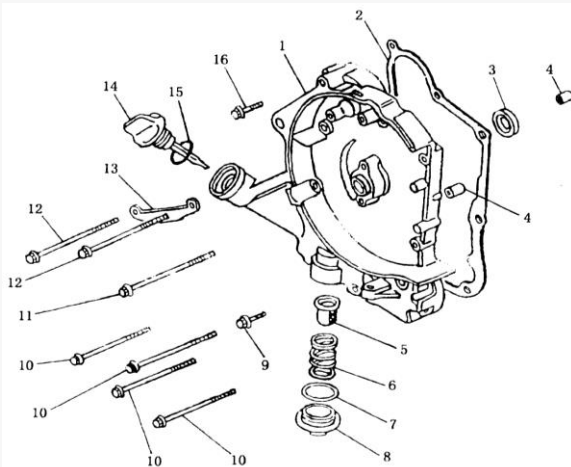
Figura N° 4: Carter
