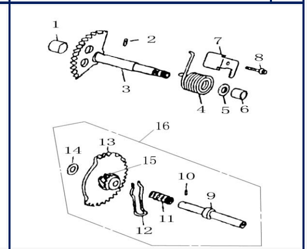
Figura N° 12: Eje de ratch
