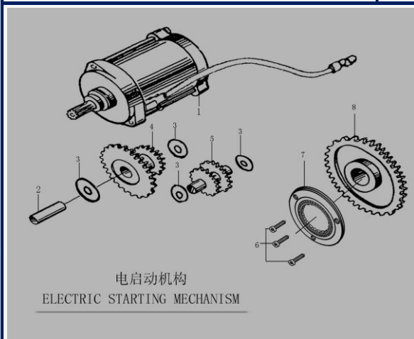
FIGURA N°28: MOTOR DE STARTER
