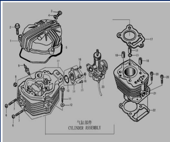
FIGURA N°18: CULATA Y CARBURADOR
