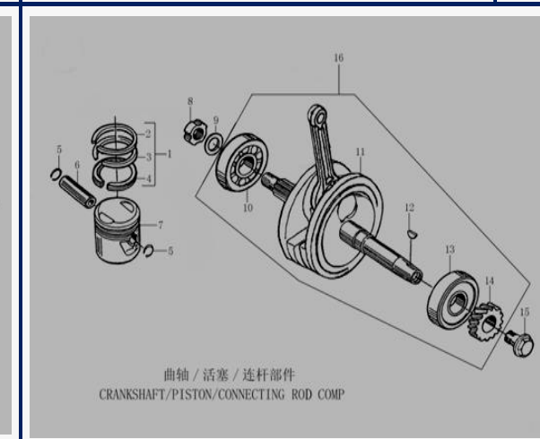
FIGURA N°24: PISTON Y CIGÜEÑAL
