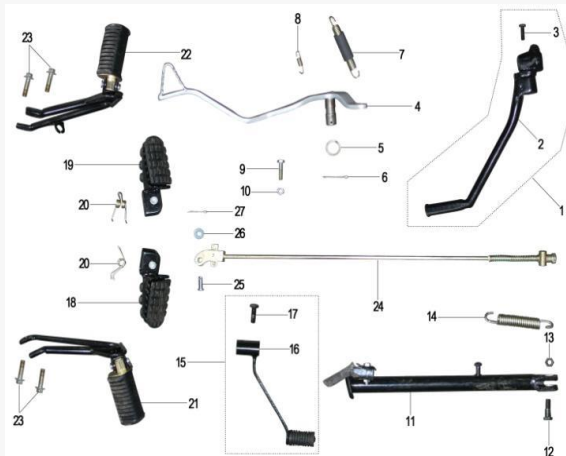
FIGURA N°16: PATA DE STARTER, VARILLA DE FRENO
