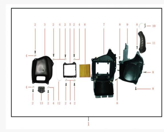
FIGURA N°12: FILTRO DE AIRE
