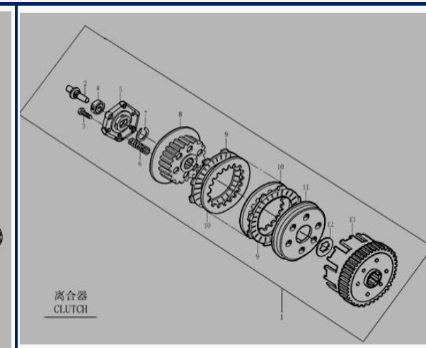
FIGURA N°21: CANASTA DE CLUTCH
