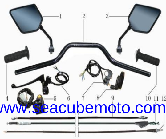
FIGURA N°2: , TIMON Y RETROVISORES
