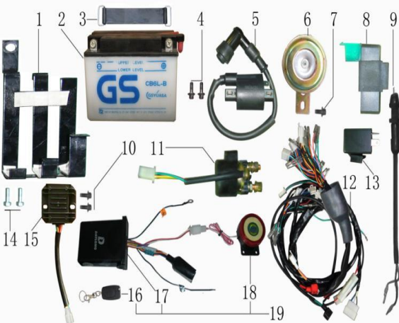
FIGURA N°17: SISTEMA ELECTRICO
