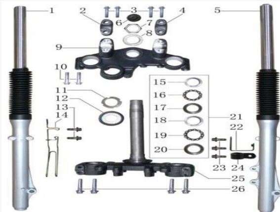
FIGURA N°3: T DE BARRAS
