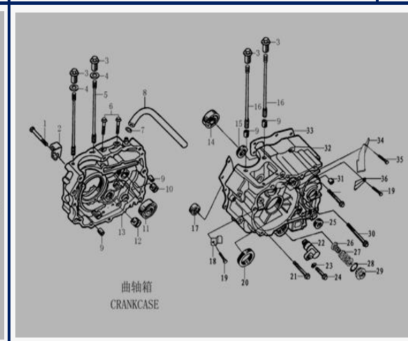
FIGURA N°23: CARTER LH
