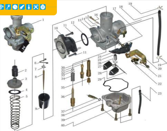
FIGURA N°13: CARBURADOR
