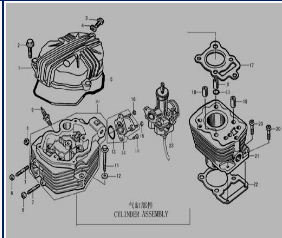
FIGURA N°18: CULATA Y CARBURADOR
