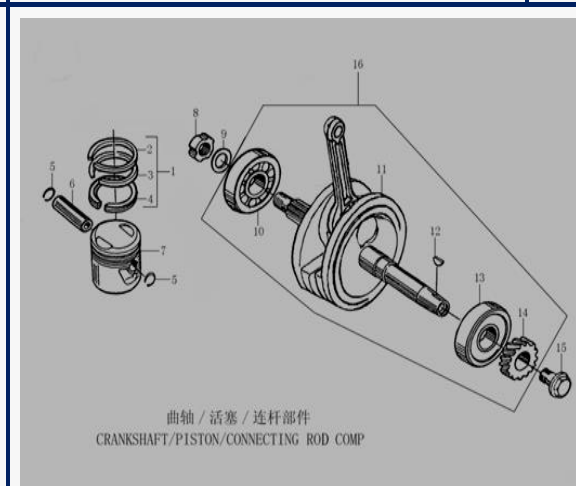
FIGURA N°24: PISTON Y CIGÜEÑAL
