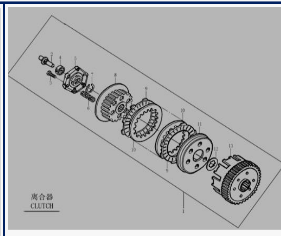
FIGURA N°21: CANASTA DE CLUTCH
