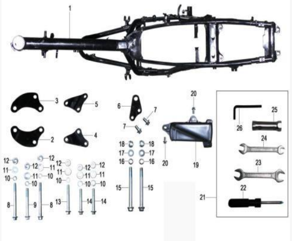
FIGURA N°9: REPOSAPIES Y COBERTRO DE TABLERO
