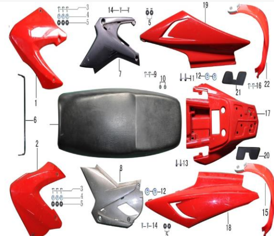
FIGURA N°15: COBERTORES DE CARROCERIA Y SILLON
