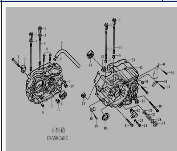
FIGURA N°23: CARTER LH
