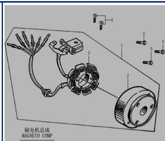
FIGURA N°27: MAGNETO
