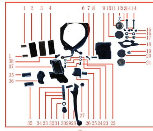
FIGURA N°5: FRENO DELANTERO
