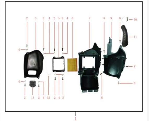
FIGURA N°12: FILTRO DE AIRE
