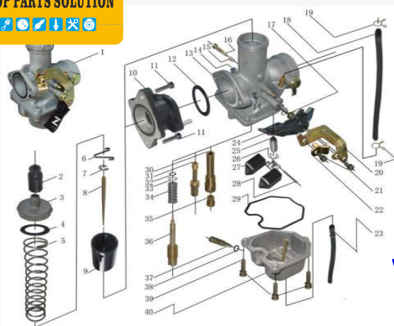
FIGURA N°13: CARBURADOR
