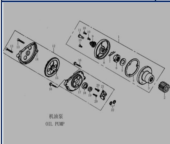
FIGURA N°22: BOMBA DE ACEITE Y FILTRO DE ACEITE
