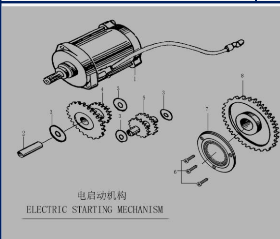
FIGURA N°28: MOTOR DE STARTER
