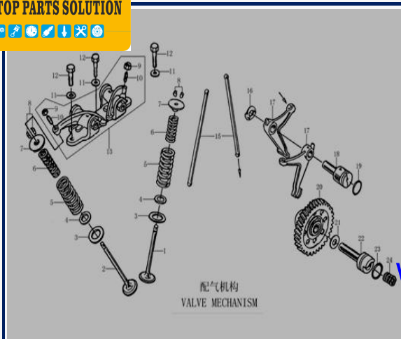
FIGURA N°19: EJE DE LEVAS Y VALVULAS
