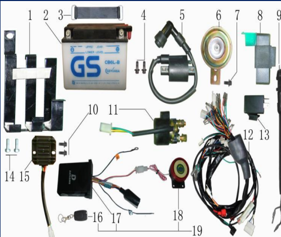
FIGURA N°17: SISTEMA ELECTRICO
