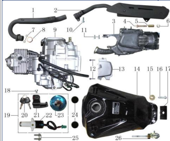
FIGURA N°10: ESCAPE Y TANQUE DE GASOLINA
