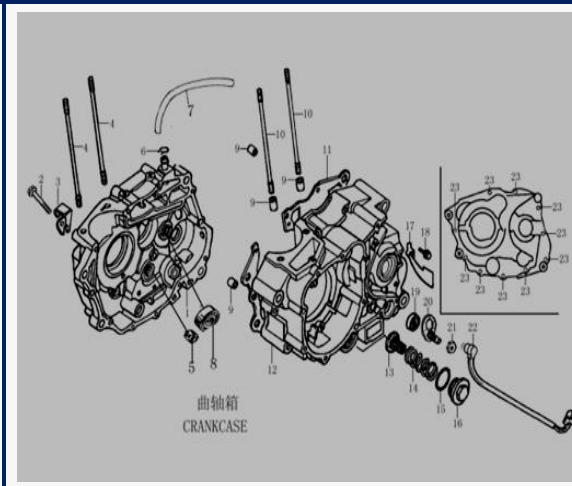
FIGURA N°23: CARTER RH
