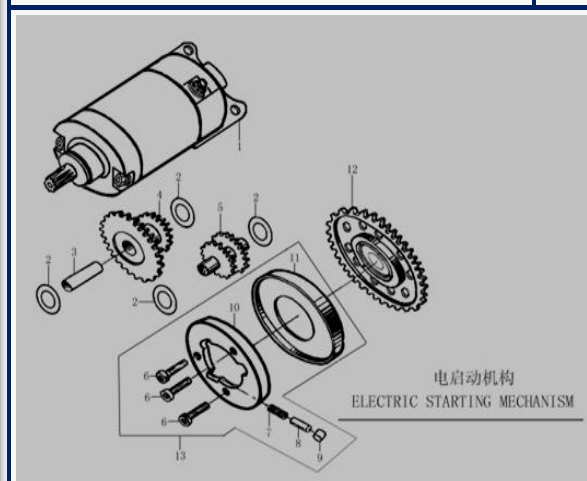
FIGURA N°28: MOTOR DE ESTARTER
