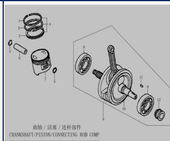
FIGURA N°24: CIGÜEÑAL Y PISTON
