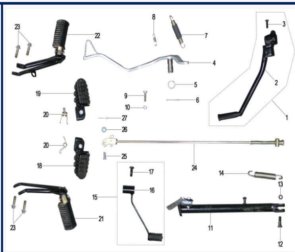
FIGURA N°15: PATA DE STARTER, VARILLA DE FRENO
