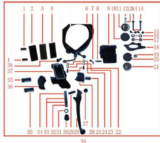
FIGURA N°5: FRENO DELANTERO
