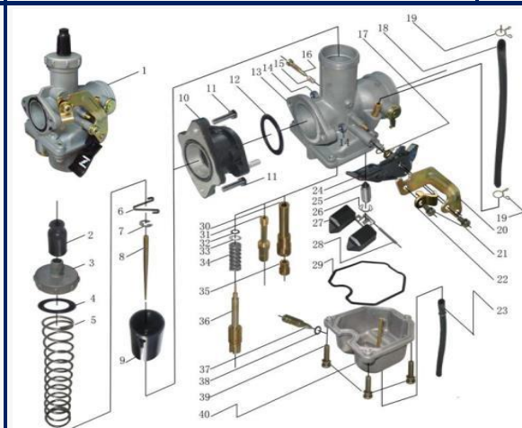
FIGURA N°12: CARBURADOR
