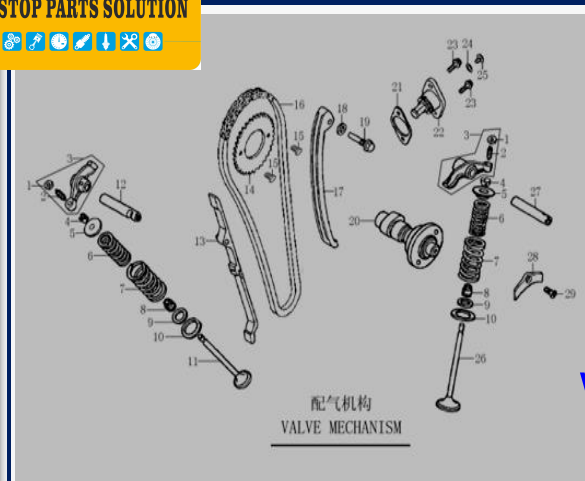
FIGURA N°19: MECANISMO DE VALVULA
