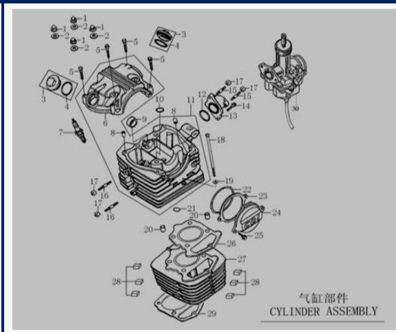
FIGURA N°18: MOTOR
