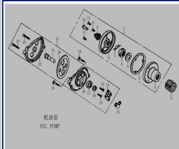
FIGURA N°22: BOMBA DE ACEITE
