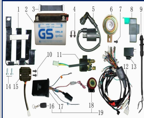
FIGURA N°16: SISTEMA ELECTRICO
