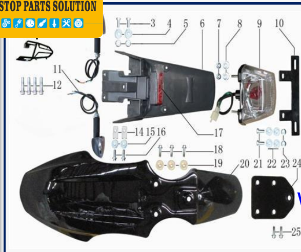
FIGURA N°13: LODERA TRASERA, LUZ DE STOP Y PIDEVIAS
