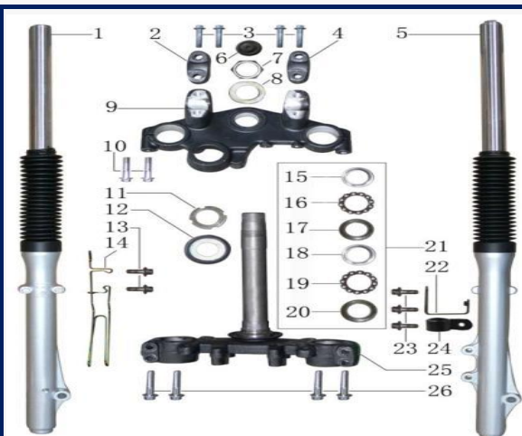
FIGURA N°3: T DE BARRAS
