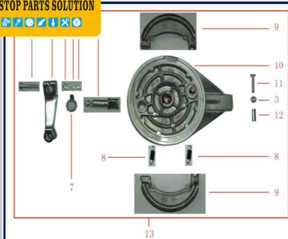
FIGURA N°7: TAMBOR DE FRENO
