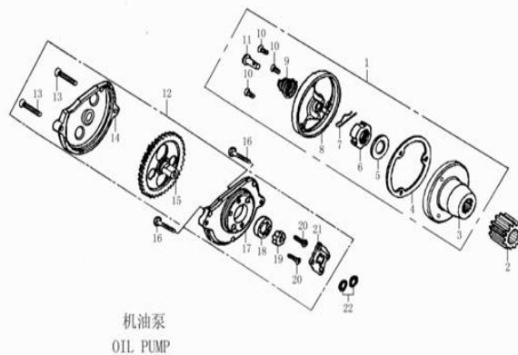
FIGURA N°22: BOMBA DE ACEITE
