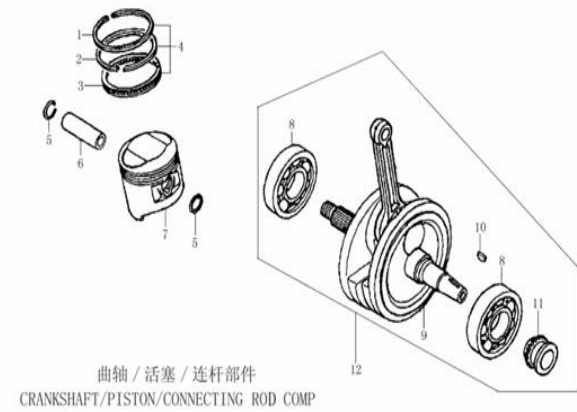
FIGURA N°24: CIGÜEÑAL Y PISTON
