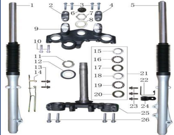
FIGURA N°3: TREN DELANTERO
