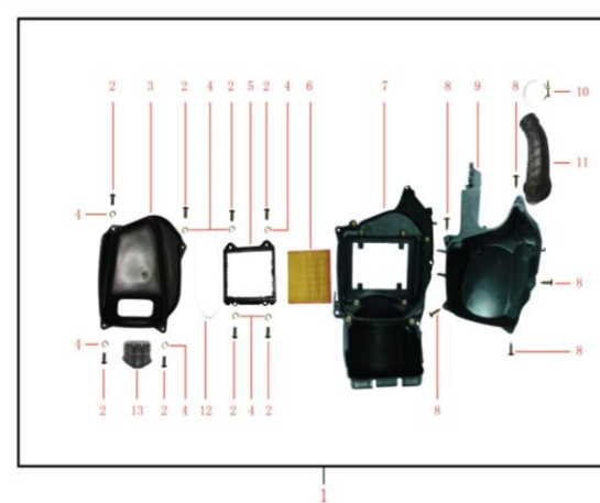
FIGURA N°11: FILTRO DE AIRE
