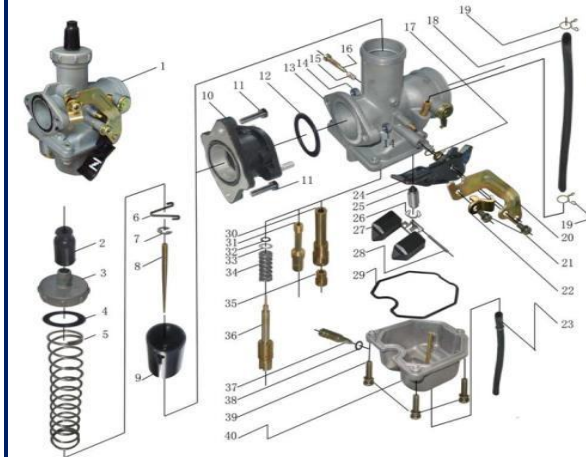
FIGURA N°12: CARBURADOR
