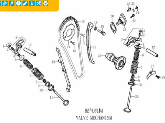
FIGURA N°19: TENSOR Y VALVULAS
