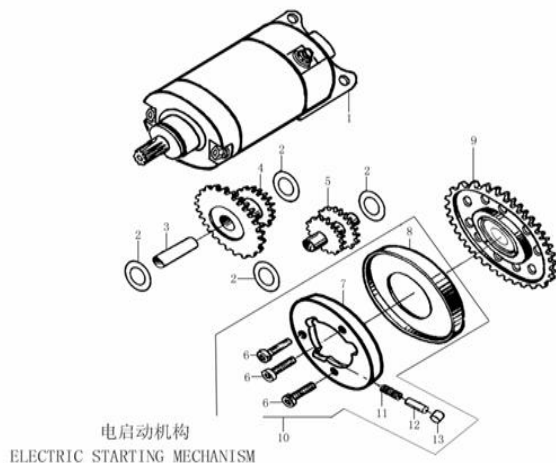
FIGURA N°28: MECANISMO DE ARRANQUE
