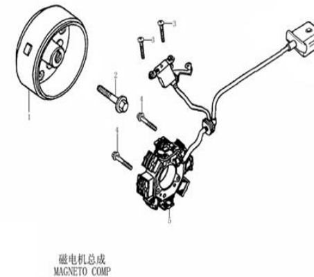
FIGURA N°27: PLANTA Y MAGNETO
