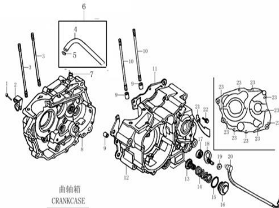
FIGURA N°23: CARTER LH Y RH
