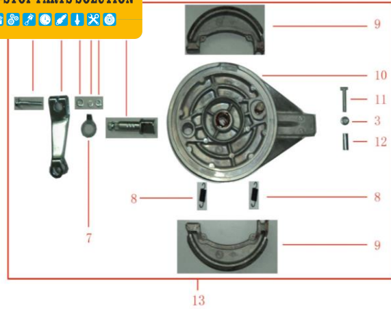
FIGURA N°7: TAMBOR DE FRENO
