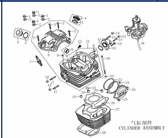
FIGURA N°18: CULATA Y CILINDRO
