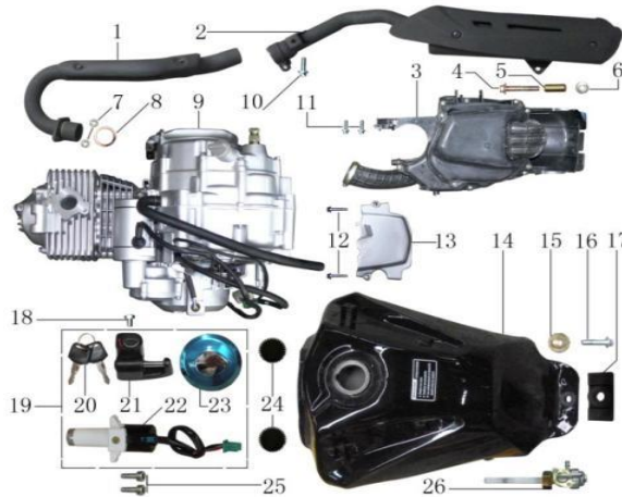
FIGURA N°10: ESCAPE, TANQUE, FILTRO Y MOTOR
