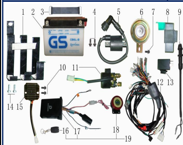
FIGURA N°16: SISTEMA ELECTRICO
