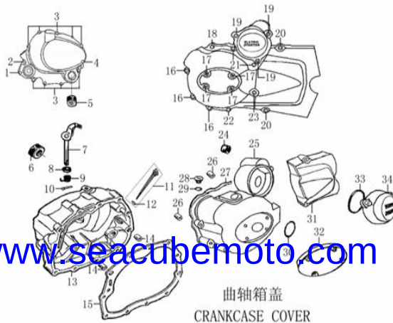
FIGURA N°20: TAPADERA DE CLUTCH Y MAGENTO
