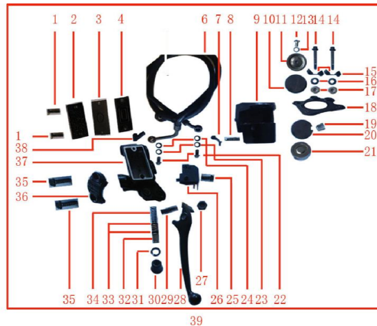
FIGURA N°5: FRENO DELANTERO
