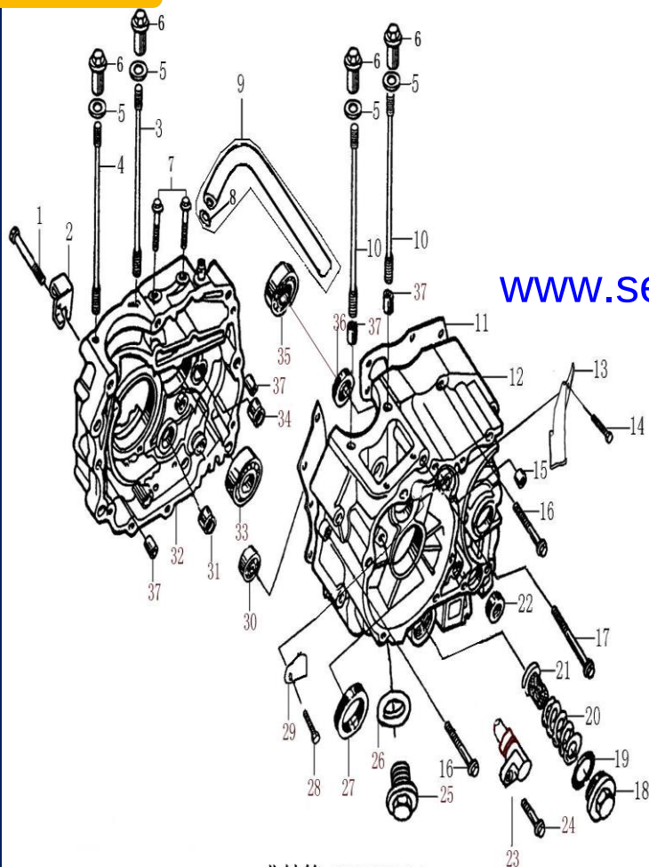
曲轴箱 CRANKCASE
