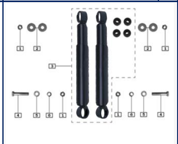
FIGURA N°30: AMORTIGUADOR
