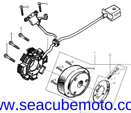
磁电机总成 MAGNETO COMP
