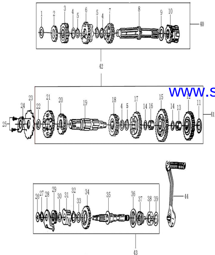
传动机构 TRANSMISSION MECHANISM
