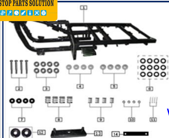
FIGURA N°7: CHASIS
