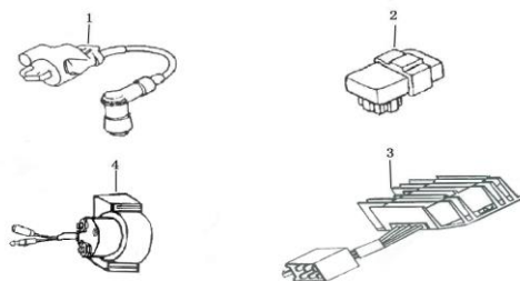
电器件 ELECTRIC
