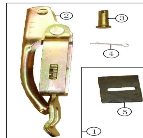
FIGURA N°12: CHAPA
