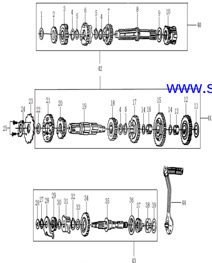
传动机构 TRANSMISSION MECHANISM
