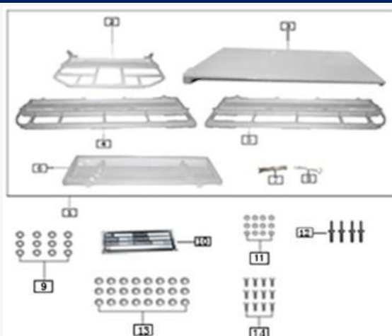
FIGURA N°11: PALANGANA
