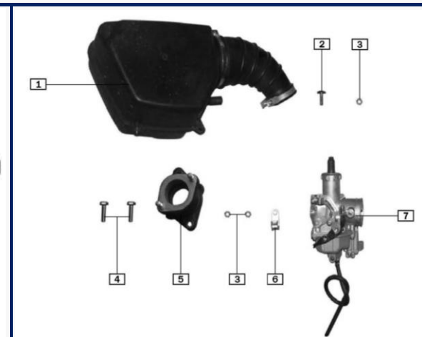
FIGURA N°3: FILTRO DE AIRE Y CARBURADOR PAG N° 3
