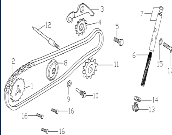
Figura N° 4: Kit de sprocket
