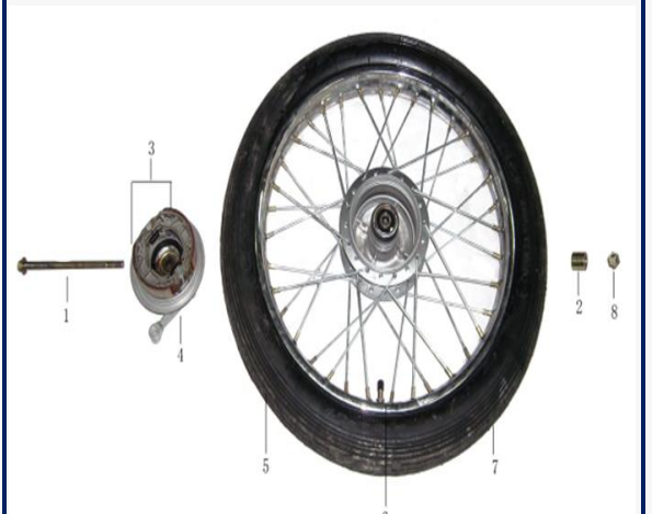
Figura N° 39: Llanta delantera
