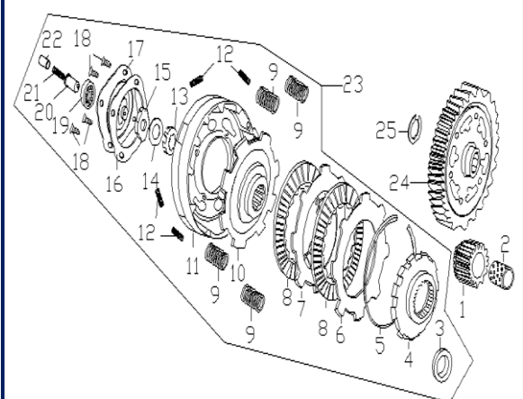
Figura N° 6: Clutch
