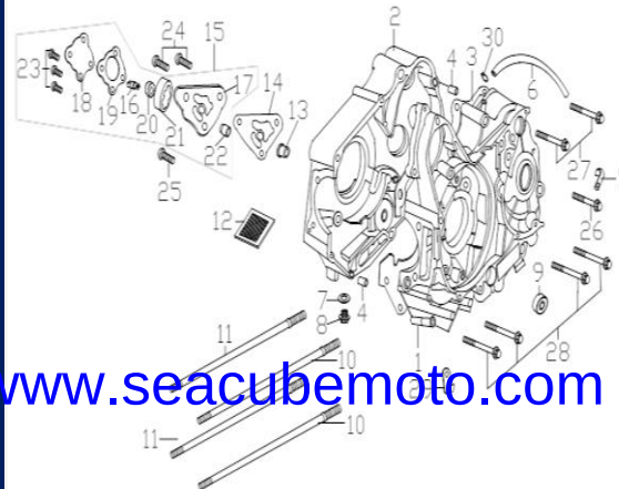
Figura N° 8: Carter
