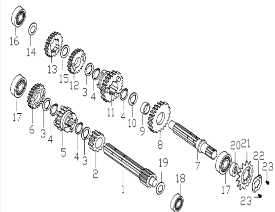
Figura N° 10: Transmision
