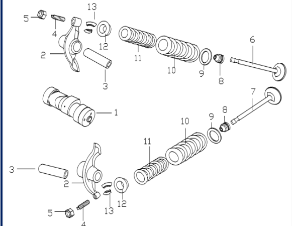
Figura N° 3: Valvulas
