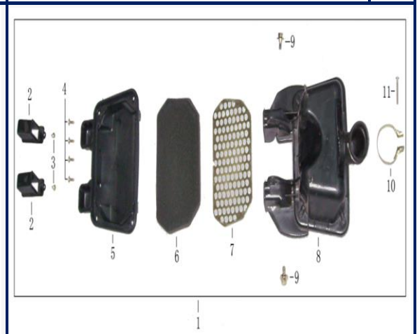
Figura N° 24: Filtro de aire
