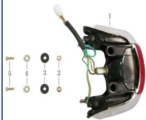
Figura N° 36: Stop
