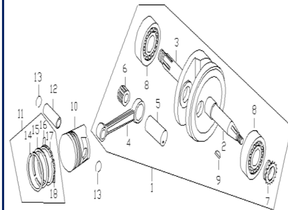
Figura N° 9: Cigüeñal
