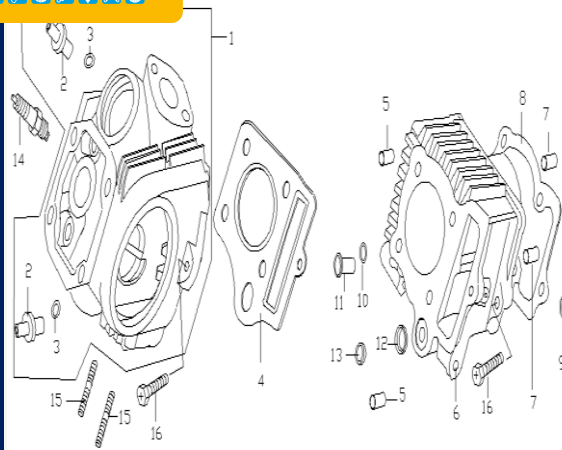
Figura N° 1: Culata
