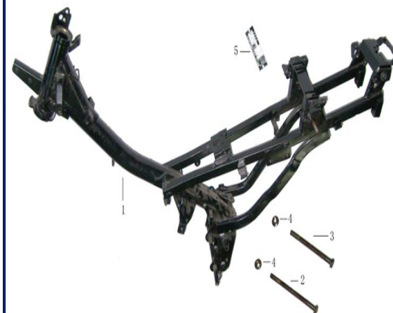
Figura N° 15: Chasis
