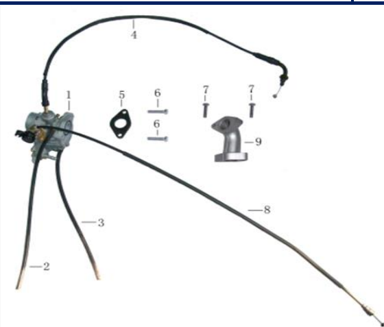
Figura N° 23: Carburador
