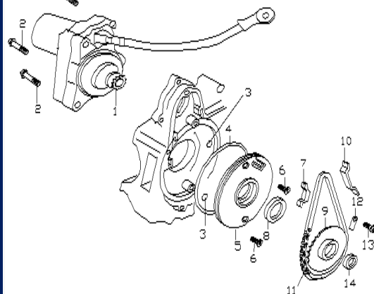
Figura N° 13: Motor de arranque
