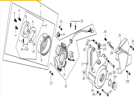
Figura N° 7: Kit de arranque
