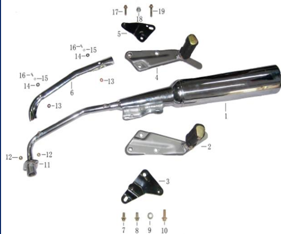
Figura N° 34: Escape
