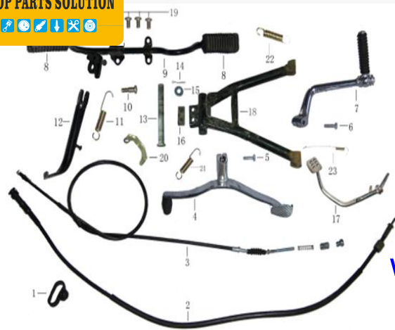
Figura N° 37: Reposapiés
