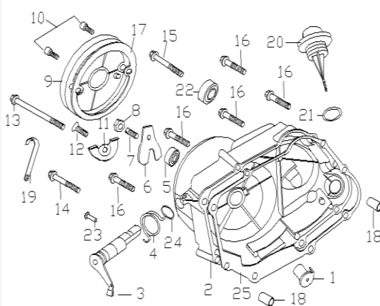
Figura N° 5: Tapadera de clutch
