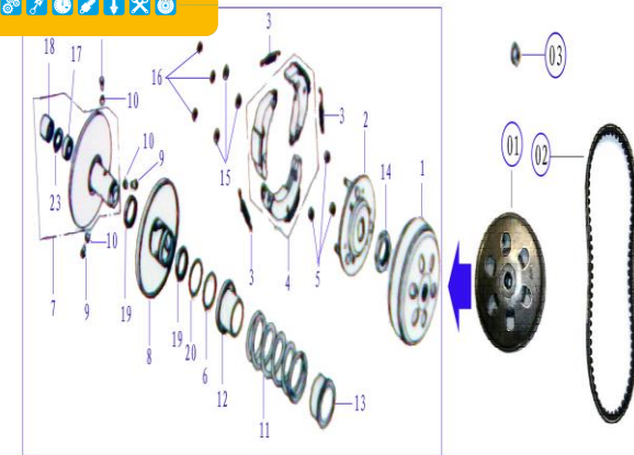
FIGURA N°13: CLUTCH COMPLETO
