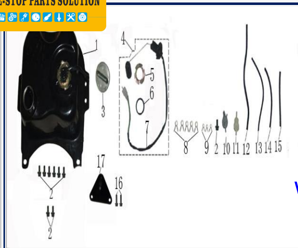
FIGURA N°25: TANQUE DE GASOLINA
