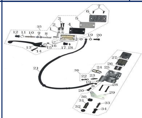
FIGURA N°29: MORDAZA DE FRENO
