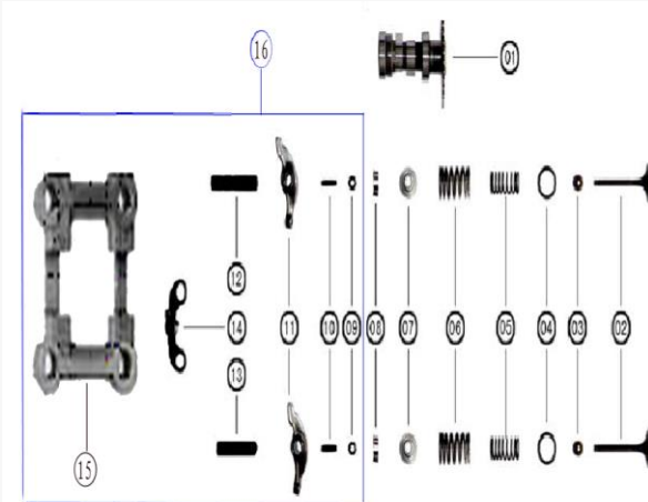
FIGURA N°3: VALVULA/EJE DE LEVAS
