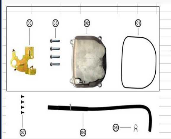
FIGURA N°5: COBERTOR DE CULATA
