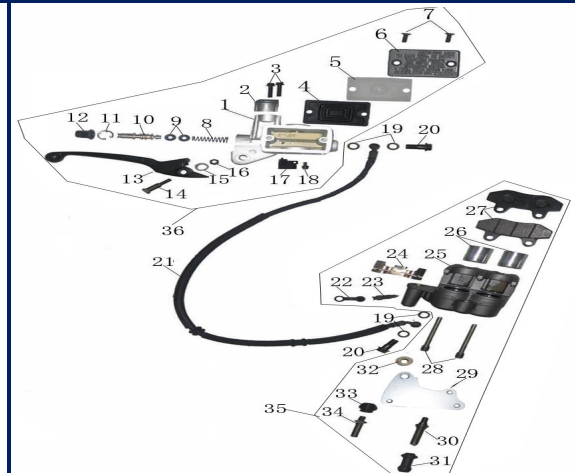
FIGURA N°30: SISTEMA DE FRENOS
