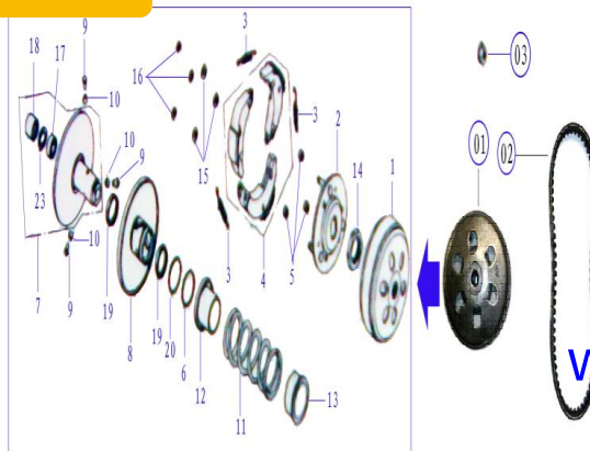
FIGURA N°13: CLUTCH COMPLETO
