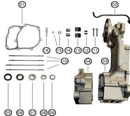
FIGURA N°15: CARTER LH
