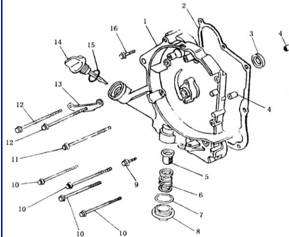
FIGURA N°23: COBERTOR COMPLETO RH
