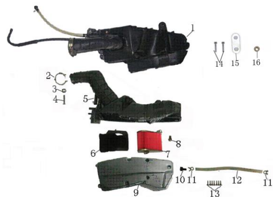
FIGURA N°16: FILTRO DE AIRE
