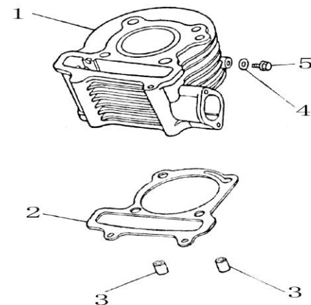
FIGURA N°24: CILINDRO
