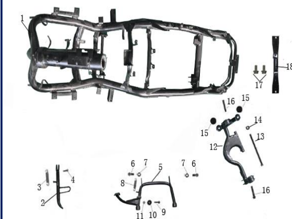
FIGURA N°15: MULETA Y AMORTIGUADOR
