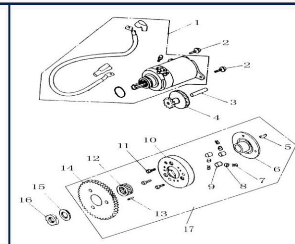
Figura N° 9: Estárter
