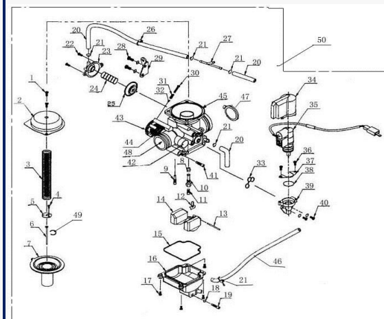
Figura N°15: Carburador
