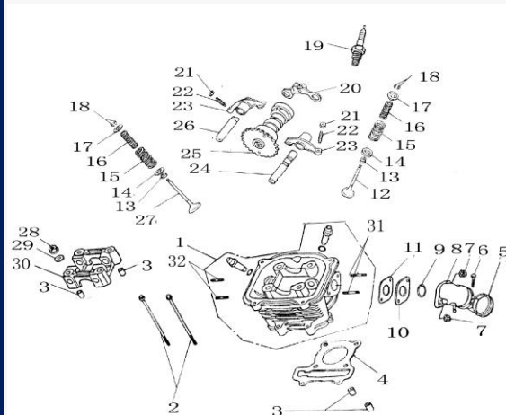
Figura N° 6: Culata
