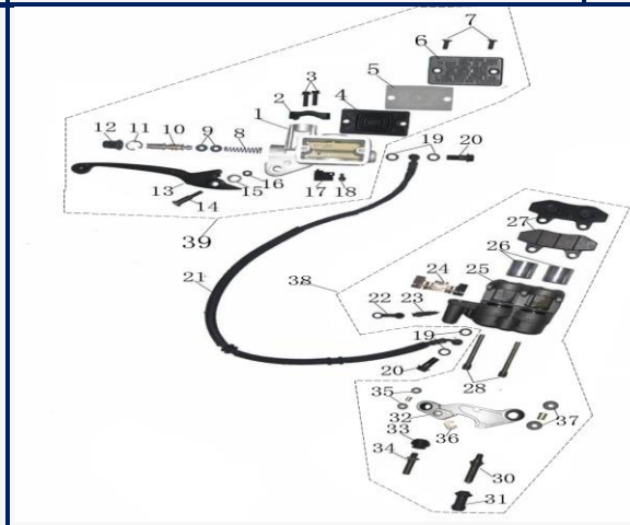
Figura N° 29: Sistema de frenos
