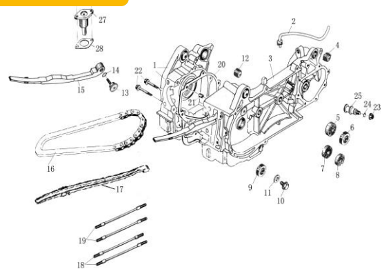
Figura N° 1: Motor
