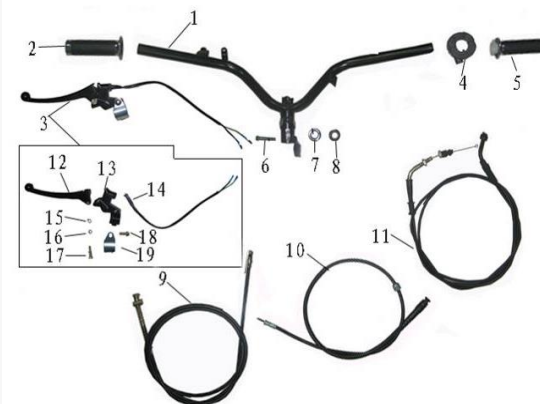
Figura N° 18: Timón
