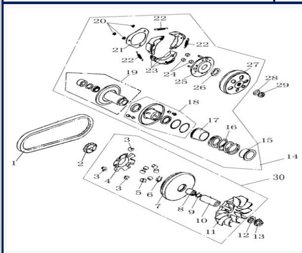
Figura N° 10: Clutch
