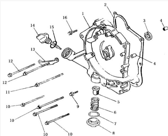
Figura N° 4: Carter
