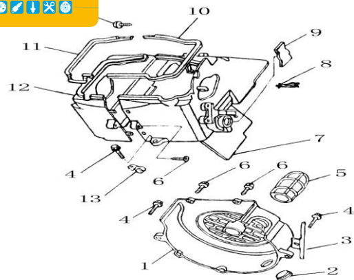
Figura N°13: Conducto de enfriamiento
