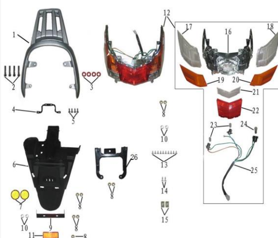
Figura N° 23: Cobertores traseros
