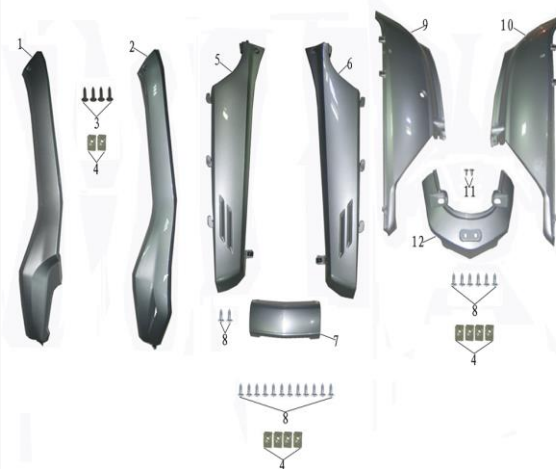
Figura N° 22: Cobertores laterales
