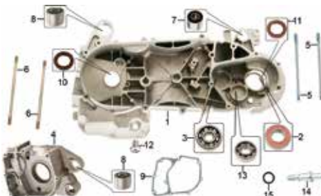
CÁRTER E-7
