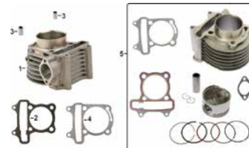
CILINDRO E-3
