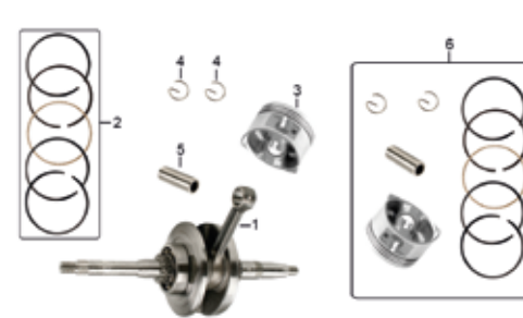
CIGÜEÑAL E-8
