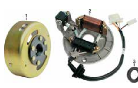
GENERADOR E-5
