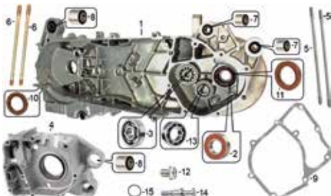
CÁRTER E-7
