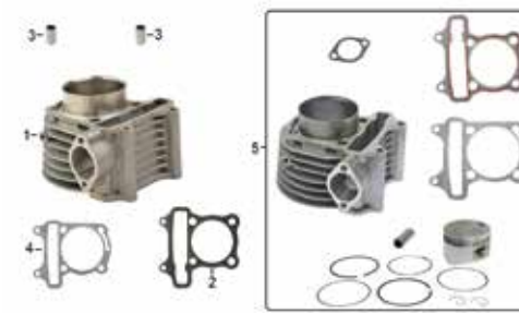
CILINDRO E-3
