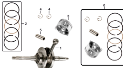
CIGÜEÑAL E-8
