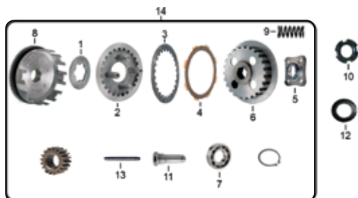
SISTEMA DE EMBRAGUE E-13
