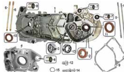
CÁRTER E-7
