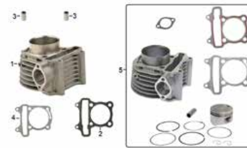
CILINDRO E-3
