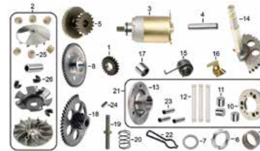
ARRANQUE E-12
