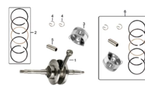
CIGÜEÑAL E-8
