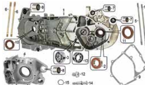
CÁRTER E-7
