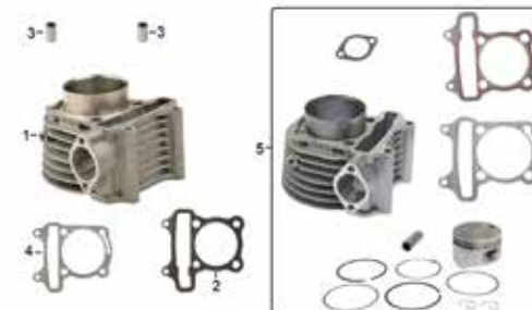
CILINDRO E-3
