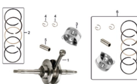
CIGÜEÑAL E-8
