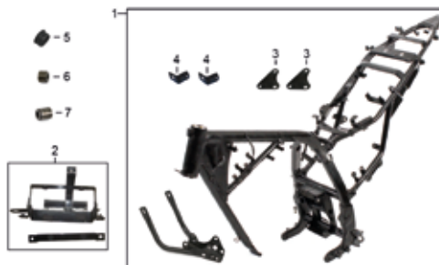
CUADRO F-5
