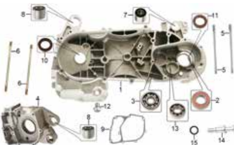
CÁRTER E-7
