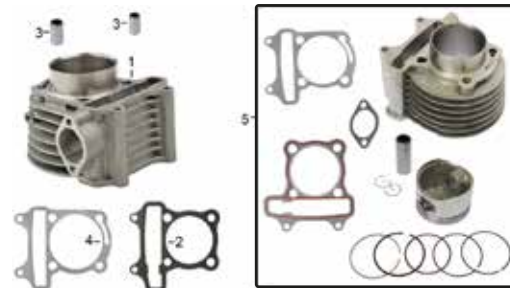
CILINDRO E-3
