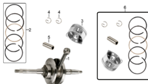
CIGÜEÑAL E-8
